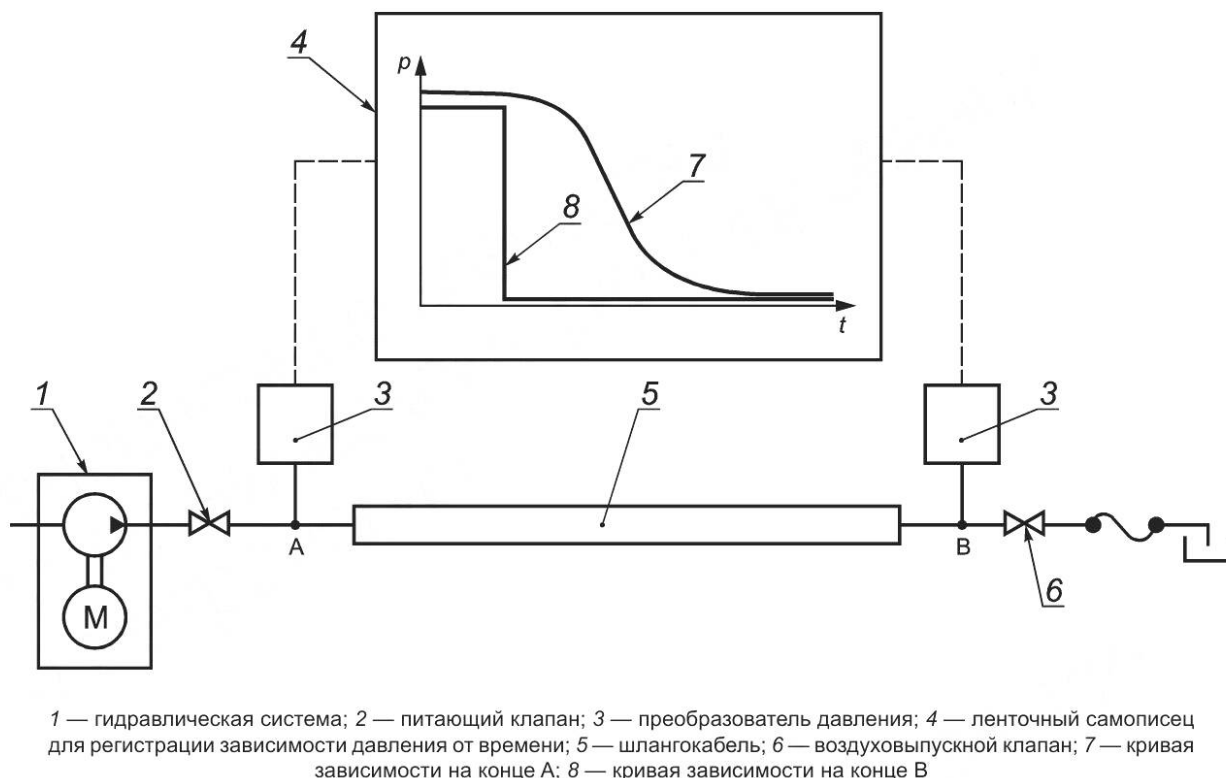
Рисунок D.2 — Схема установки для проведения динамических испытаний полимерных труб
