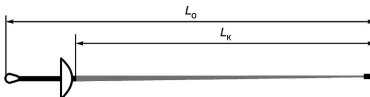
Рисунок 1 — Схема фехтовального спортивного снаряда
