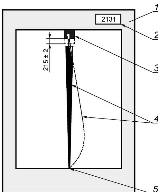
Рисунок 2 — Схема измерения жесткости прогиба клинка рапиры и шпаги
