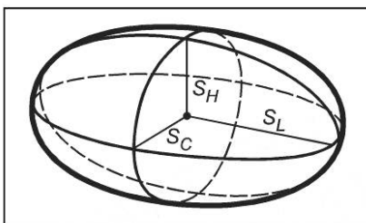
Рисунок 2 — Трехмерное пространство допусков CMC
