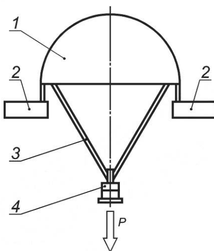
Рисунок 5 — Стенд для испытания подбородочного ремня противоударного шлема
