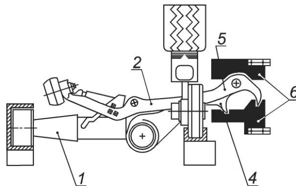
б — контроль положения подвижной и неподвижной губок зажима перед зацеплением
