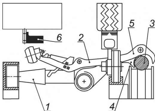
а — контроль взаимного положения ролика подвижного рычага зажима после отцепления
