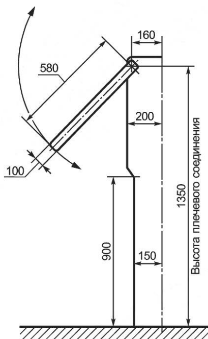
Рисунок Б.4 — Устройство для определения расположения поручней и опор для рук
