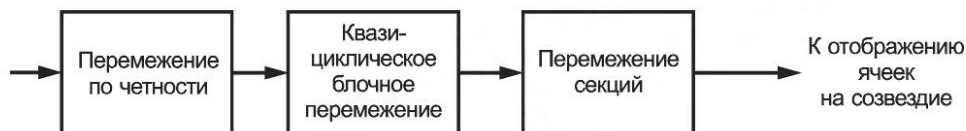
Рисунок 6 — Структурная схема битового перемежителя профиля MIMO
