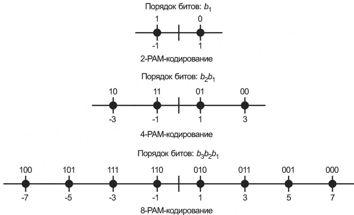
Рисунок 10 — Битовое кодирование и маркировка реальных символов РАМ
