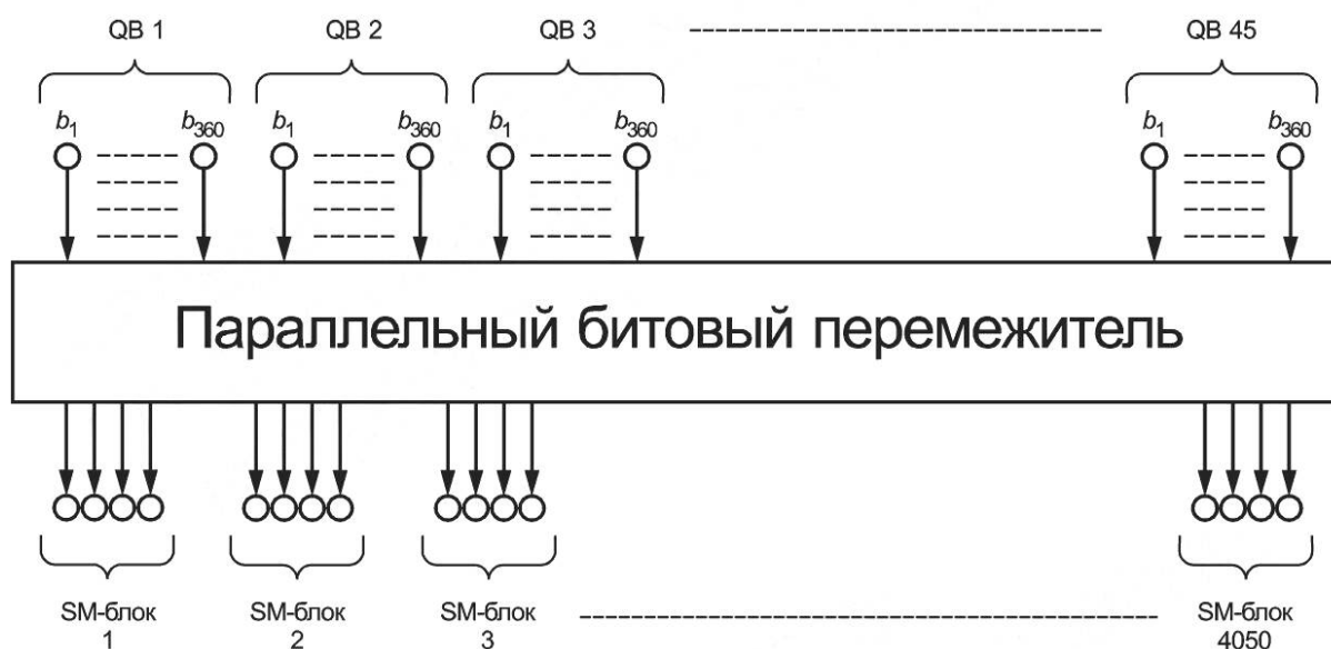
Рисунок 7 — Структурная схема параллельного битового перемежителя для N_{bpsu} = 8
