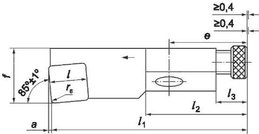
б) Для резцов-вставок высотой h_1 = 10, 12, 16 и 20 мм высотой
