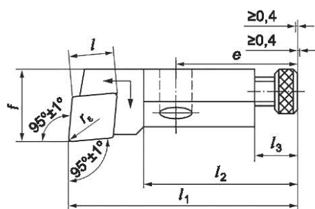
а) Для резцов-вставок высотой h_1 = 6, 8, 10, 12, 16 и 20 мм
