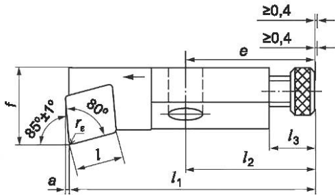
а) Для резцов-вставок высотой h_1 = 6 и 8 мм
