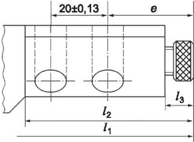
в) Для резцов-вставок h_1 = 25 мм
