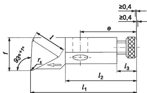
а) Для резцов-вставок высотой h_1 = 8, 10, 12, 16 и 20 мм
