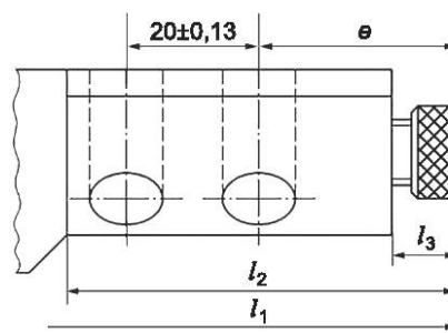
б) Для резцов-вставок высотой h_1 = 25 мм
