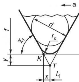
Рисунок 30 — Главный угол в плане \chi_r \leq 90^\circ с продольной подачей
