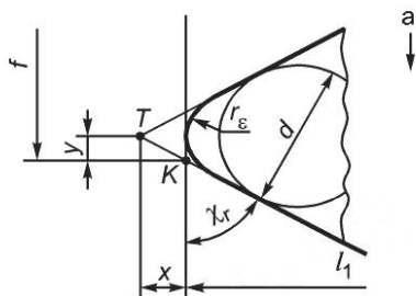
Рисунок 29 — Главный угол в плане \chi_r \leq 90^\circ с поперечной подачей
