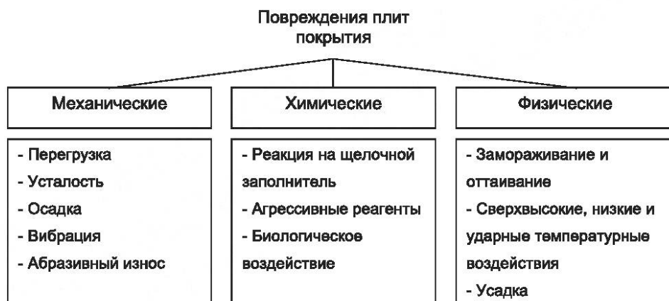
Рисунок 1 — Классификация причин повреждения бетона
