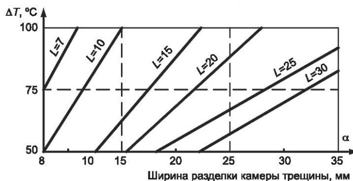
Рисунок Б.1 — Номограмма для определения ширины разделки камеры трещины при использовании герметика с предельным относительным удлинением 50 % при температуре минус 20 ^\circ\text{C}
