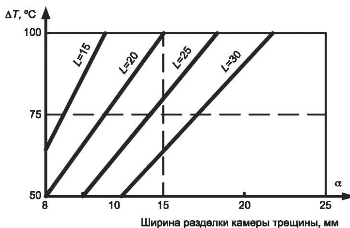
Рисунок Б.3 — Номограмма для определения ширины разделки камеры трещины при использовании герметика с предельным относительным удлинением 150 % при температуре минус 20 ^\circ\text{C}
