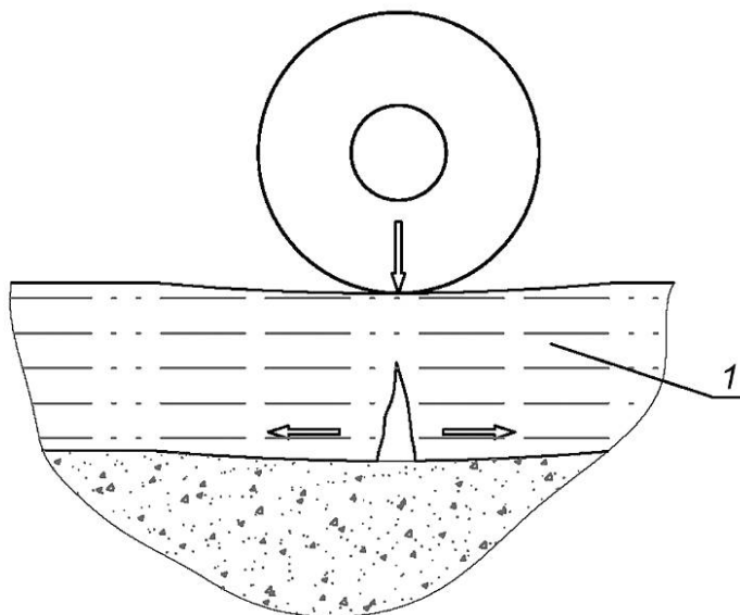
Рисунок А.2 — Схема образования силовой трещины
