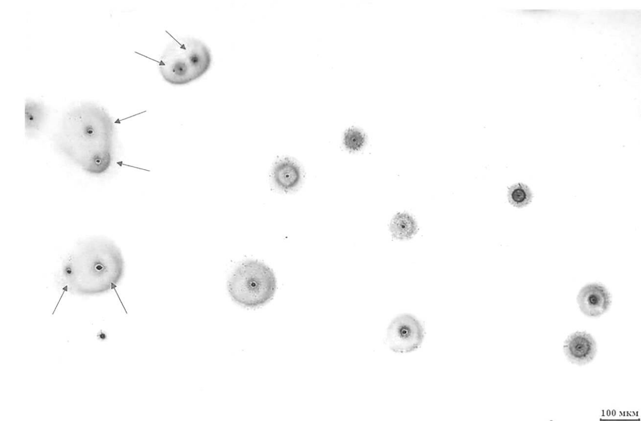
б — пример 2 двух близкорасположенных КАНВ 2-го типа в левой части снимков шлифа, которые пересекаются/соприкасаются своими гало [при подсчете учитывают как два отдельных КАНВ 2-го типа (показано стрелками)]
