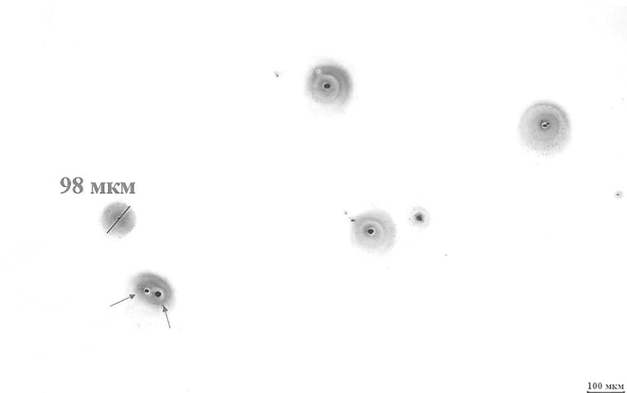
а — пример 1 двух близкорасположенных КАНВ 2-го типа в левой части снимков шлифа, которые пересекаются/соприкасаются своими гало [при подсчете учитывают как два отдельных КАНВ 2-го типа (показано стрелками)]. Пример 1 измерения размера гало КАНВ 2-го типа
