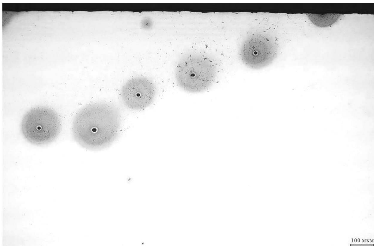
в — пример изображения КАВВ 2-го типа
