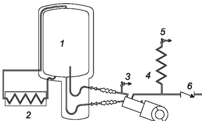
1 — резервуар хранения; 2 — испаритель наддува (PBU); 3 — предохранительный клапан на стороне всасывания насоса; 4 — компенсатор пульсаций; 5 — предохранительный клапан подачи; 6 — невозвратный клапан
