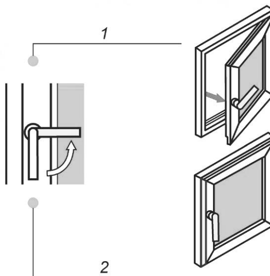
Рисунок В.1 — Оконный блок с поворотным открыванием
