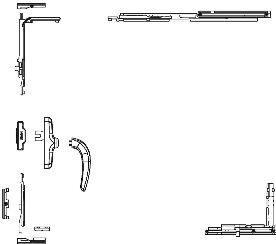
Рисунок Д.1 — Вариант съемной ручки с защелкивающимся механизмом для алюминиевых конструкций
