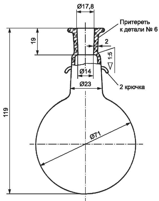
Рисунок Б.7 — Приемная колба
