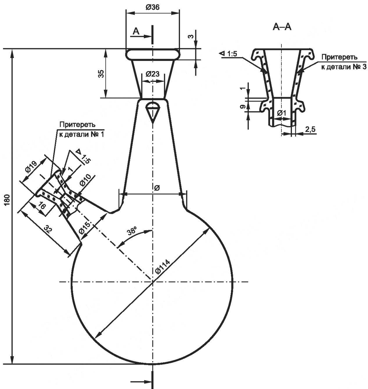
Рисунок Б.2 — Колба для перегонки
