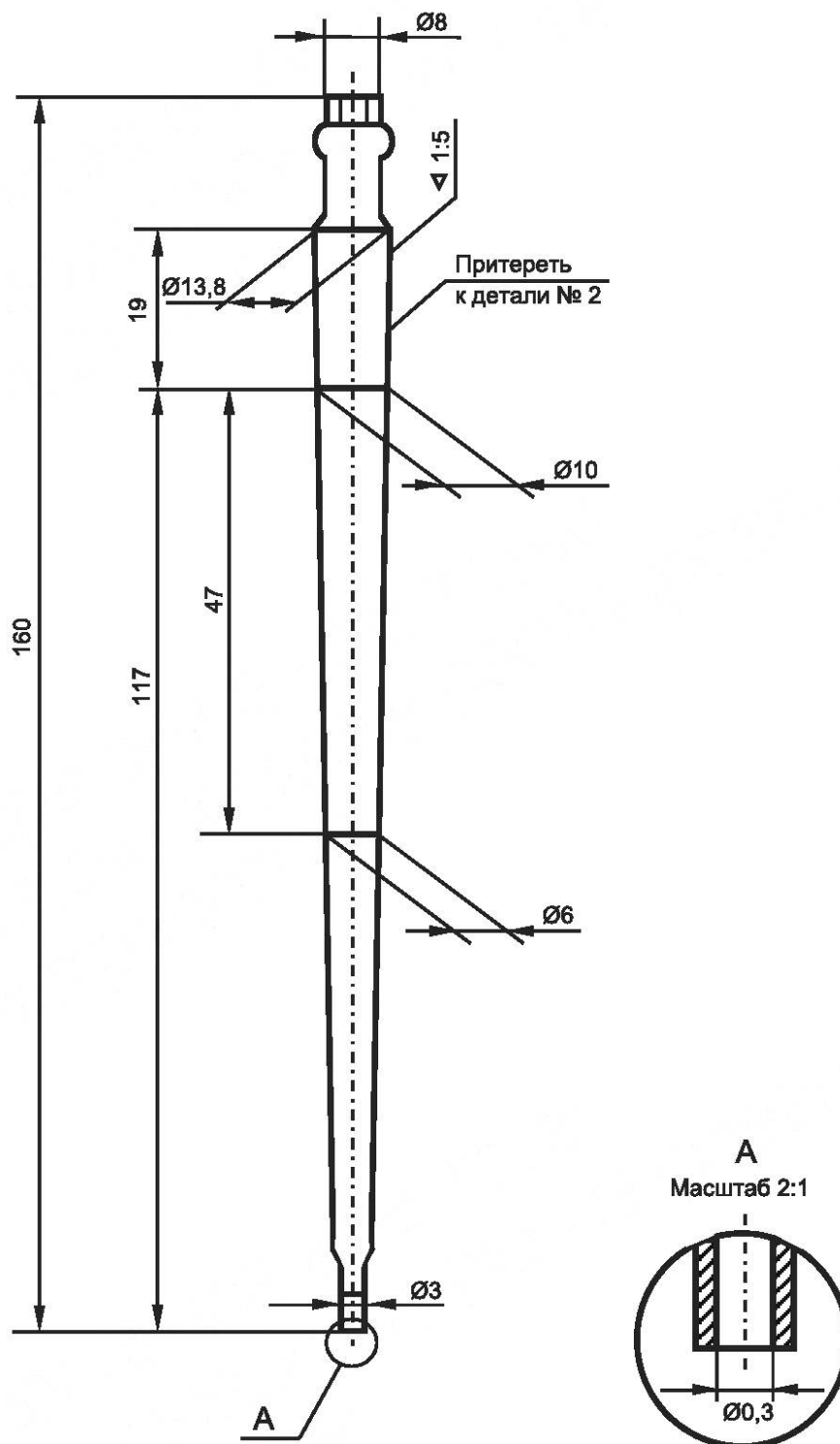
Рисунок Б.1 — Трубка капиллярная
