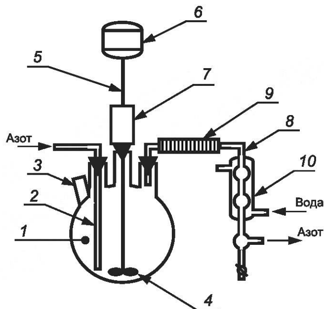
1 — четырехгорлая колба; 2 — ввод для азота; 3 — карман для термометра; 4 — мешалка с лопастью из фторопласта; 5 — ось мешалки; 6 — электродвигатель; 7 — затвор ртутный или глицериновый; 8 — соединительная трубка; 9 — асбестовый шнур; 10 — холодильник-ловушка
