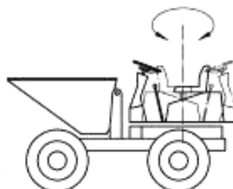
Рисунок 25 — Сиденье с круговым поворотом
