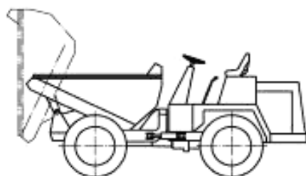
Рисунок 4 — Передняя разгрузка
