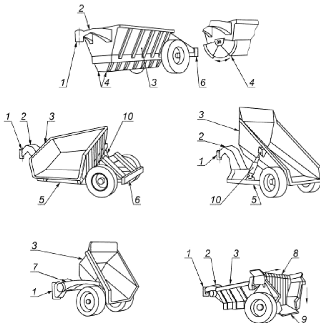
1 — подшипник поворотного шкворня; 2 — гусек; 3 — кузов; 4 — створки; 5 — основная рама; 6 — бампер; 7 — тяговая рама; 8 — выталкиватель; 9 — задний откидной борт; 10 — гидроцилиндр разгрузки
