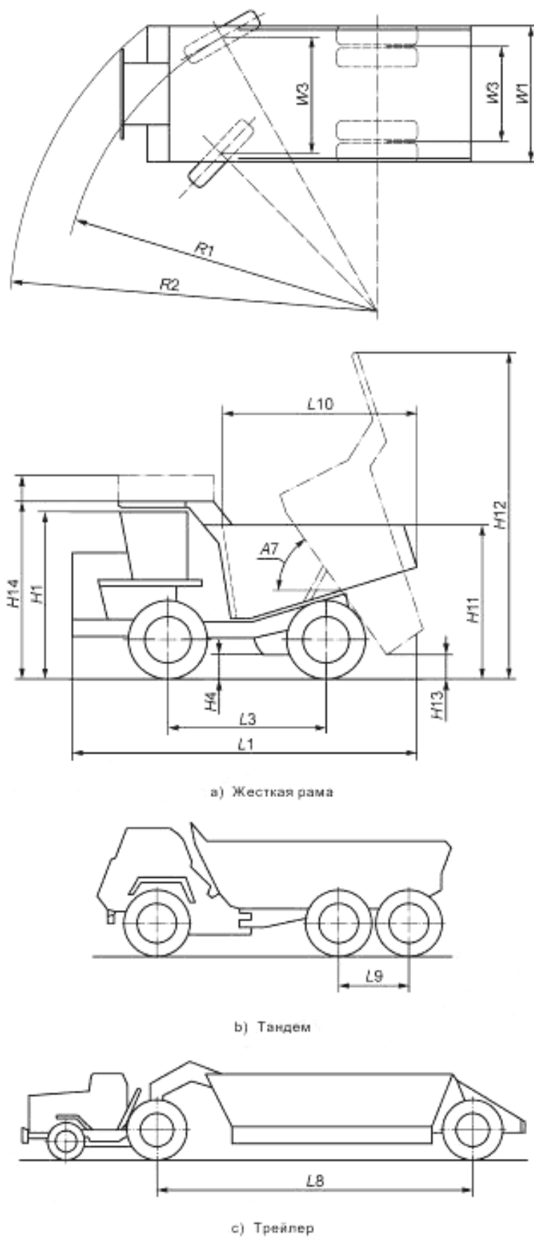
Рисунок 26 — Размеры базовой машины. Землевоз
