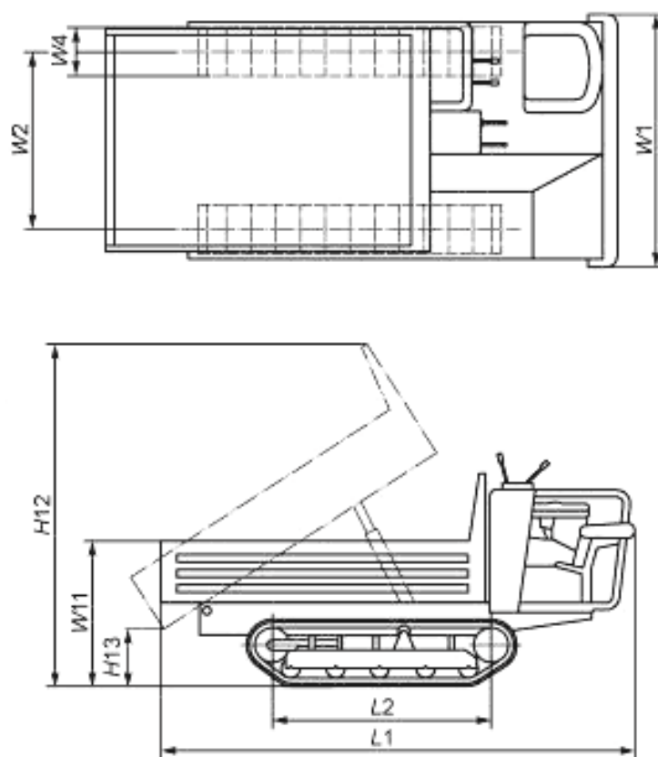
Рисунок 29 — Размеры гусеничного мини-землевоза. Сиденье сзади кузова
