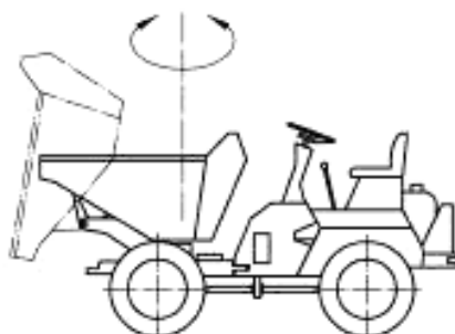
Рисунок 5 — Разгрузка с поворотом на две стороны
