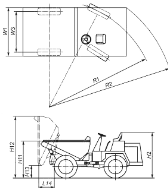
Рисунок 27 — Размеры четырехколесного мини-землевоза
