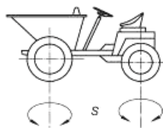
S — управляемые колеса
