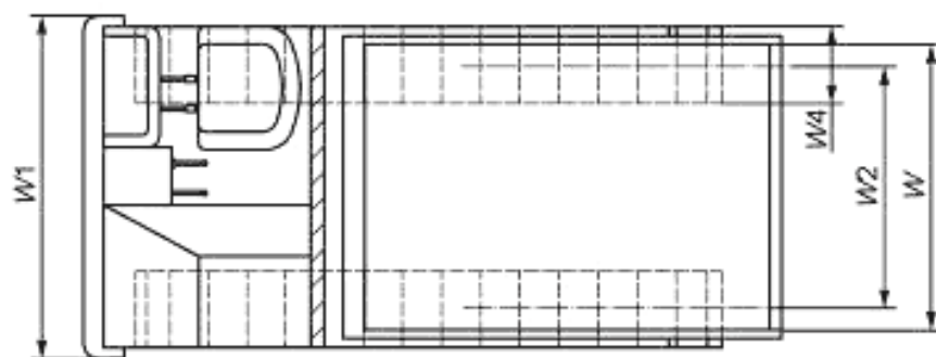
Рисунок 30 — Размеры гусеничного мини-землевоза. Сиденье спереди кузова (лист 1)
