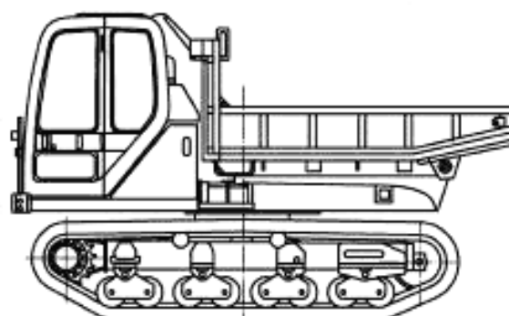
Рисунок 7 — Разгрузка с поворотной платформы землевоза
