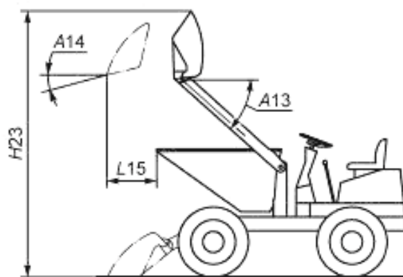
Рисунок 31 — Размеры самозагружающегося мини-землевоза
