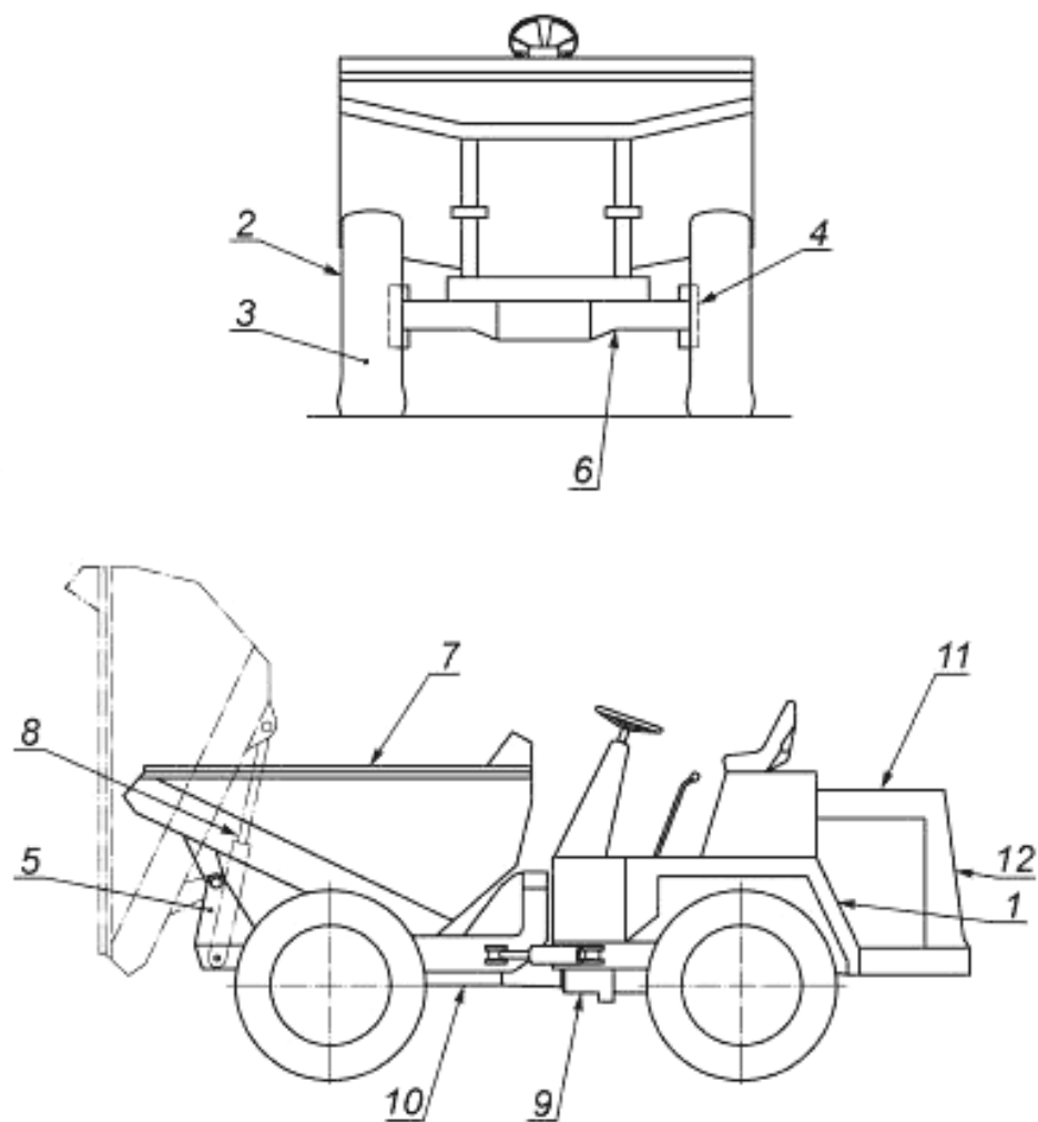
1 — крыло; 2 — колесо; 3 — шина; 4 — тормоз; 5 — ось и корпус шарнира; 6 — ось (оси); 7 — кузов; 8 — гидроцилиндр; 9 — трансмиссия; 10 — основная рама; 11 — капот; 12 — энергетическая установка
