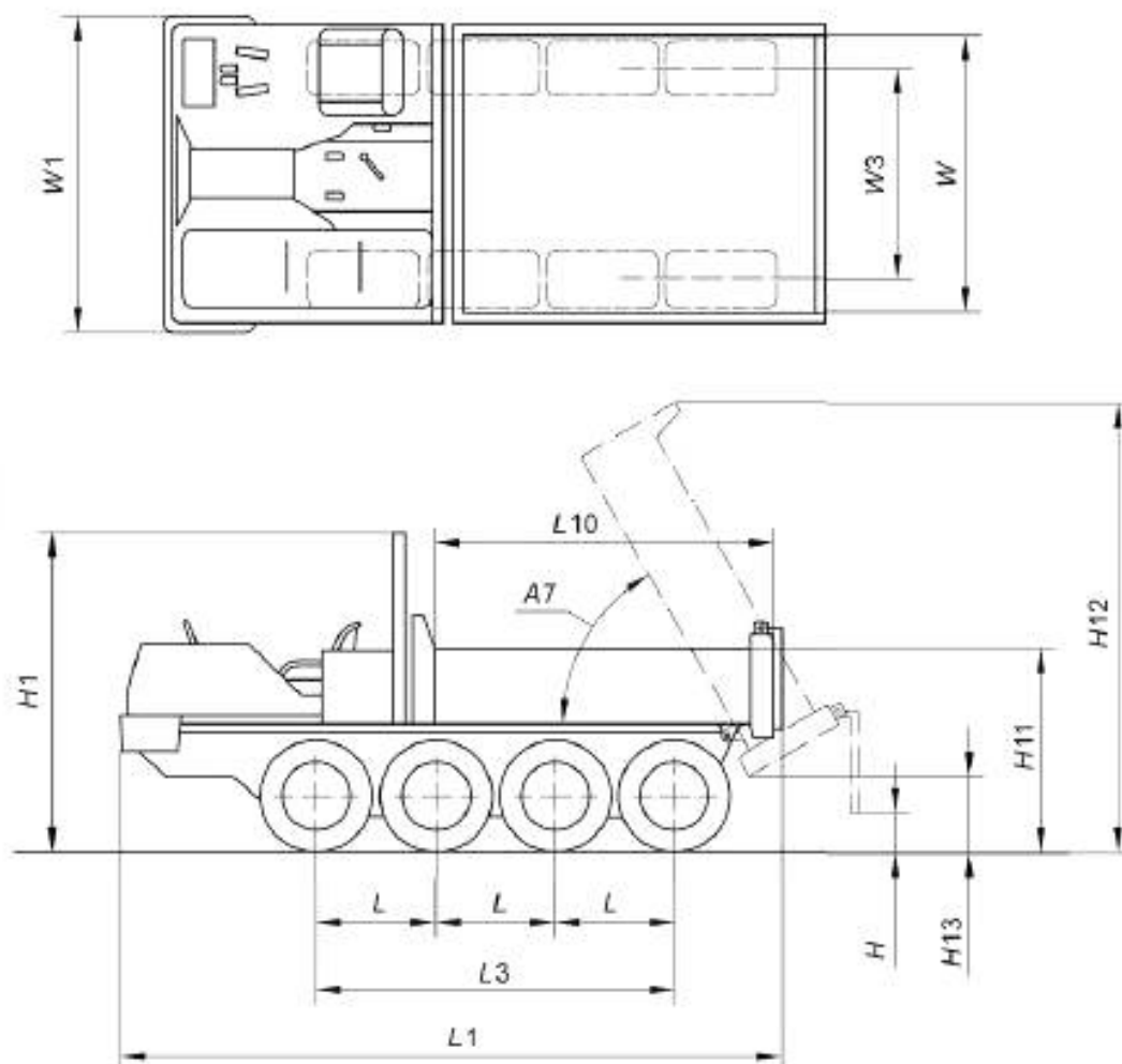
Рисунок 28 — Размеры восьмиколесного мини-самосвала
