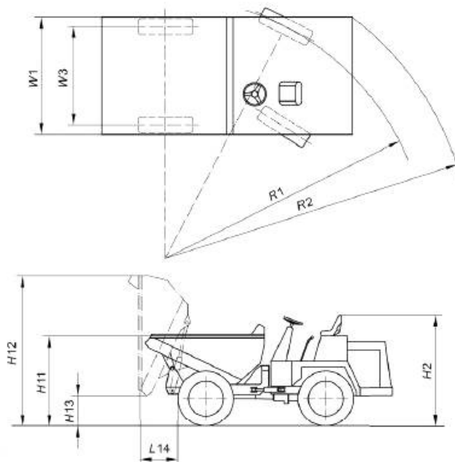
Рисунок 27 — Размеры четырехколесного мини-самосвала
