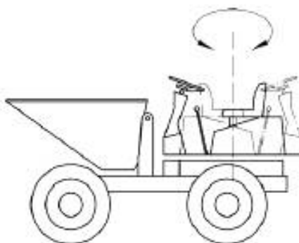
Рисунок 25 — Реверсивное рабочее место оператора
