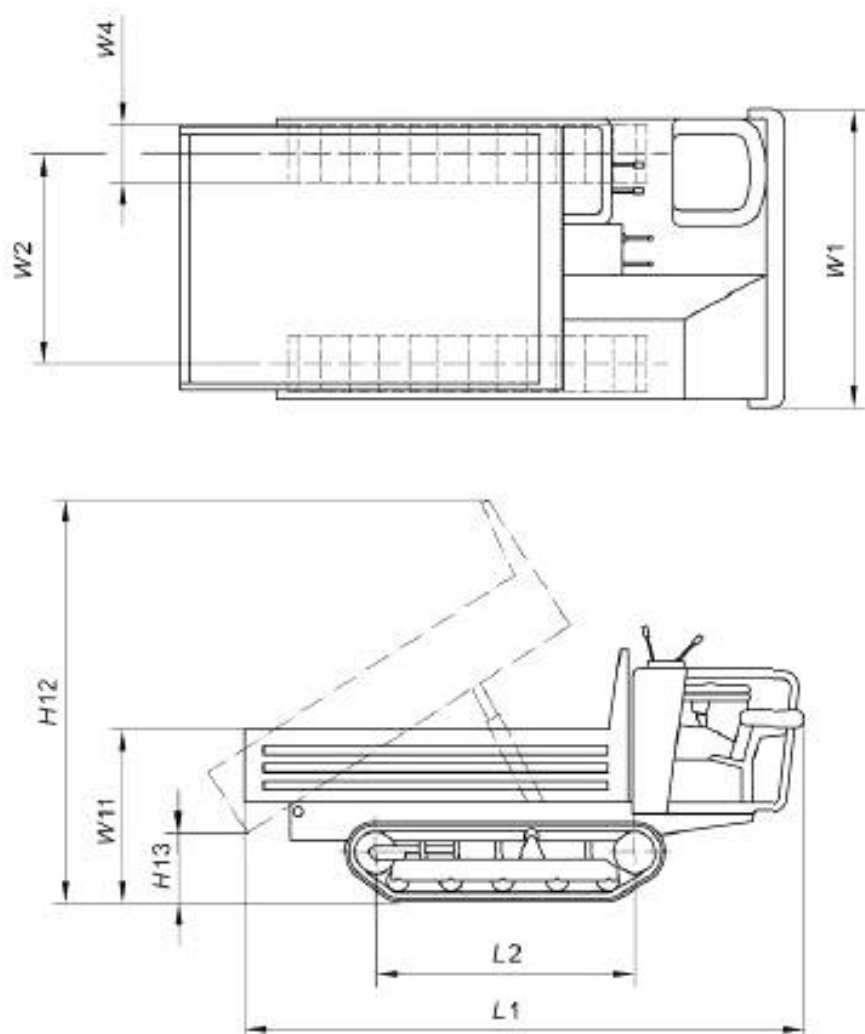
Рисунок 29 — Размеры гусеничного мини-самосвала. Рабочее место оператора сзади
