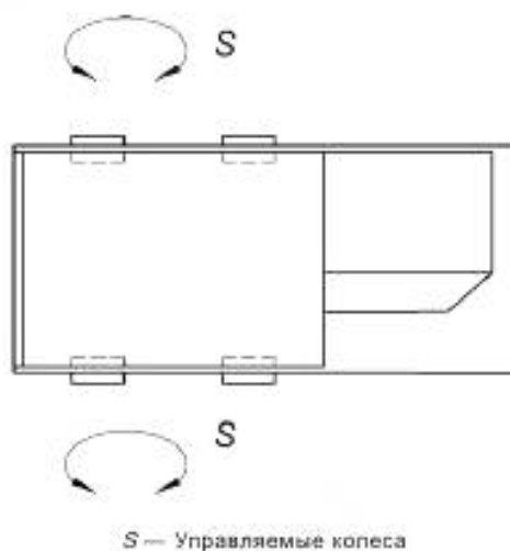
Рисунок 13 — Управление бортами с колесным двигателем
