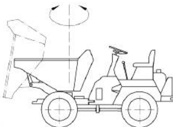
Рисунок 5 — Поворотная разгрузка
