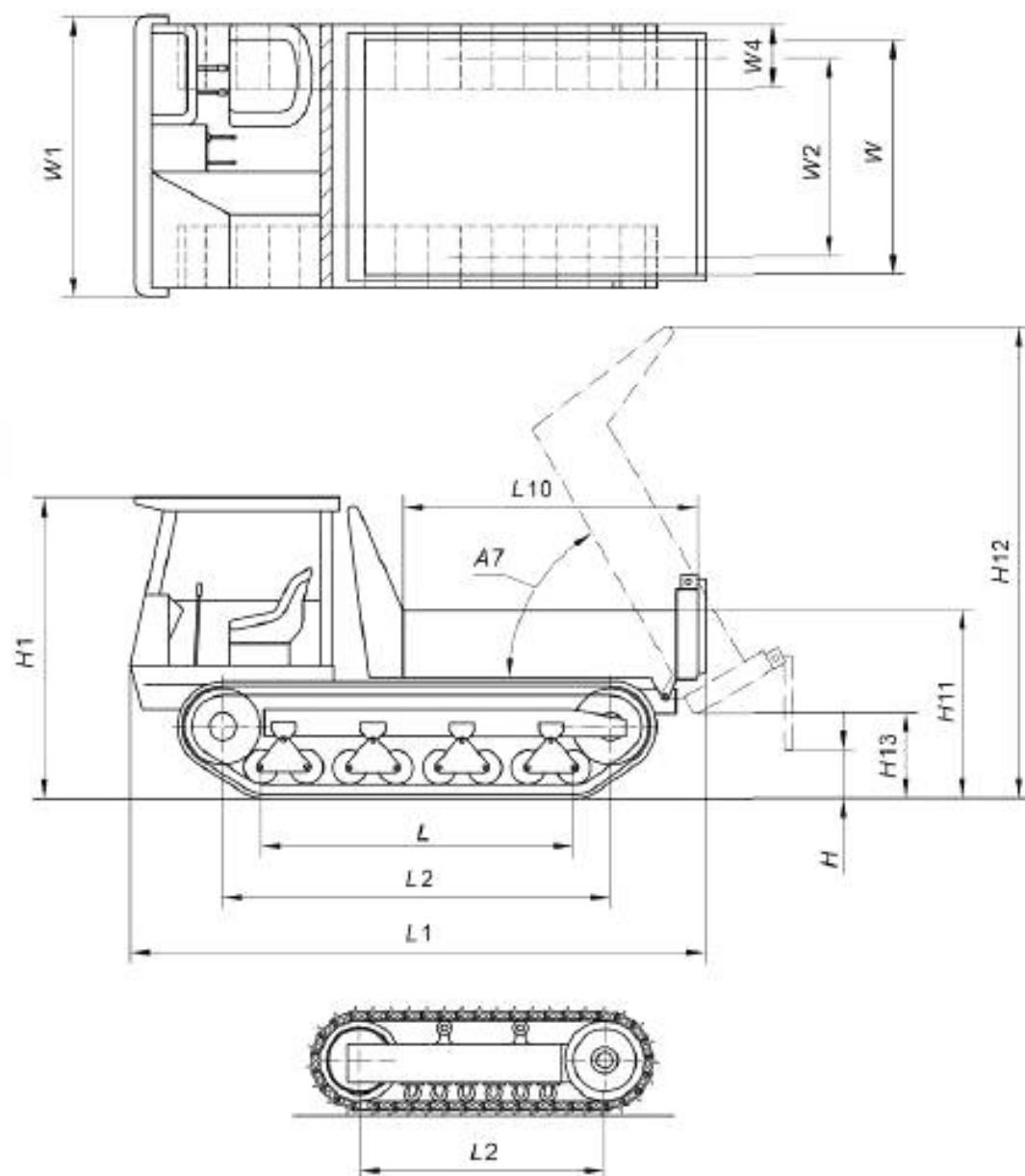
Рисунок 30 — Размеры гусеничного мини-самосвала. Рабочее место оператора спереди
