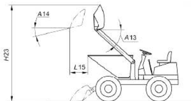
Рисунок 31 — Размеры мини-самосвала с самозагрузкой
