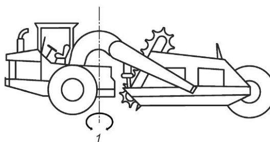
Рисунок 4 — С поворотом одноосного тягача
