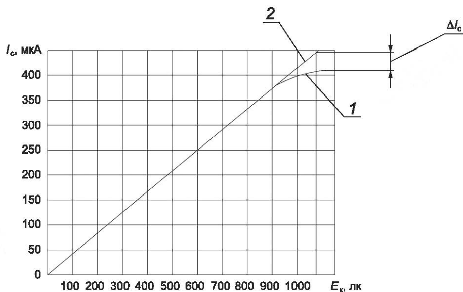
1 — световая характеристика; 2 — прямая, проведенная через точки световой характеристики
