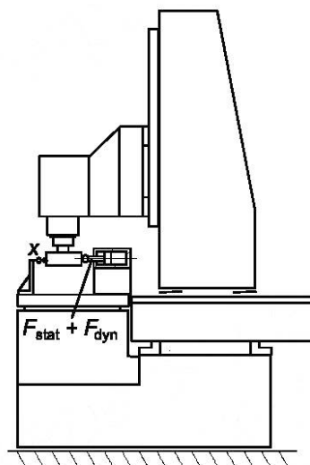
а) Возбуждение относительной вибрации
