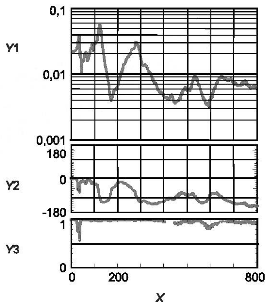
б) Частотная характеристика
