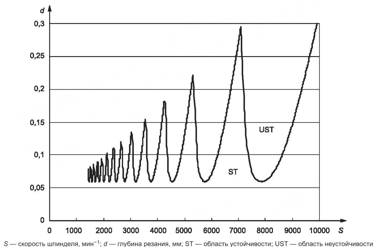
Рисунок 24 — Диаграмма устойчивости
