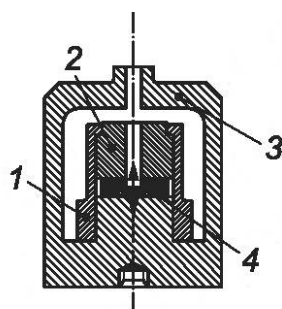
1 — втулка для создания предварительного нагружения; 2 — масса; 3 — корпус; 4 — пьезоэлемент
