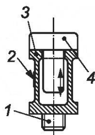
1 — резьбовая шпилька; 2 — тензометр; 3 — корпус из легкого металла; 4 — масса
