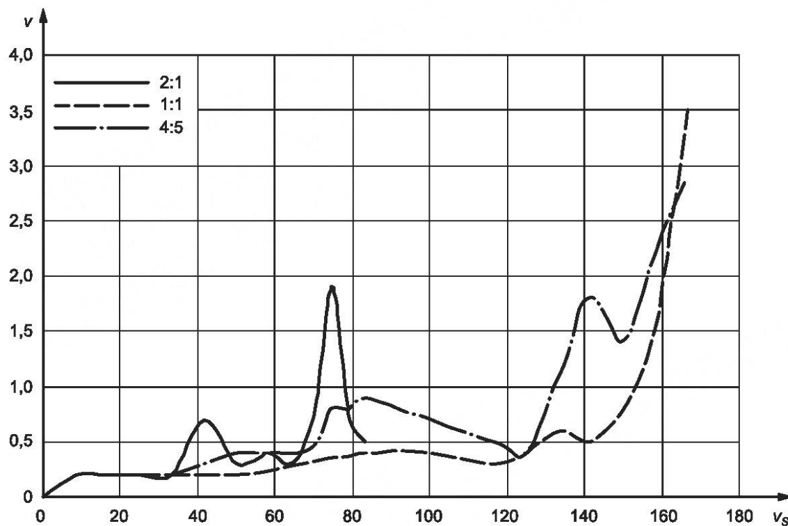
Рисунок Е.4 — Вибрация шпинделя при трех значениях передаточного числа
