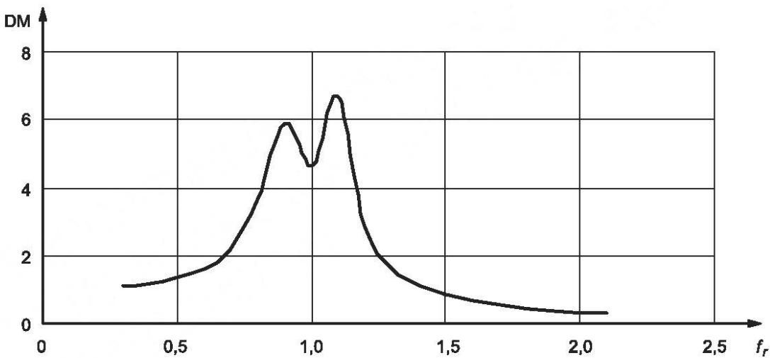
f_r — относительная частота; DM — коэффициент динамического усиления
