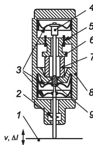
1 — вибрирующая поверхность; 2 — щуп; 3 — диафрагменные пружины; 4 — направляющий болт; 5 — катушка; 6 — полюсный наконечник; 7 — постоянный магнит; 8 — корпус; 9 — соединение с щупом; v — скорость вибрации поверхности
