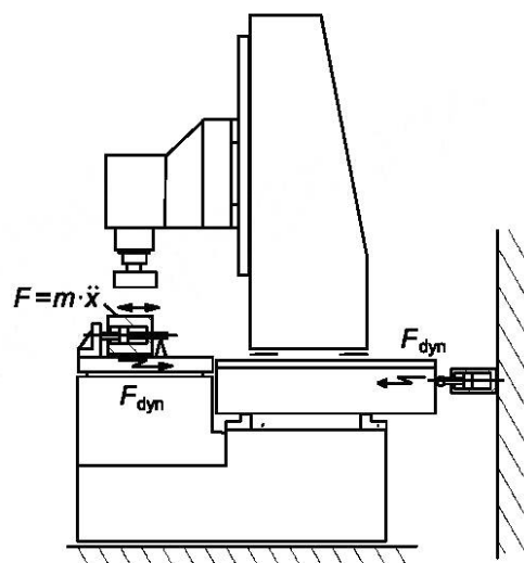
б) Возбуждение абсолютной вибрации
