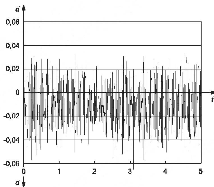
а) Вибрация в направлении X
