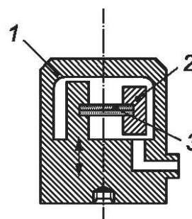
1 — корпус; 2 — масса; 3 — пьезоэлемент
