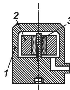
1 — корпус; 2 — масса; 3 — пьезоэлемент
