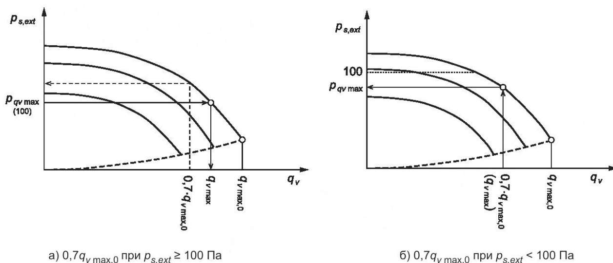
Рисунок Г.1 — Примеры оценки максимального объемного расхода воздуха и давления для агрегата категории D
