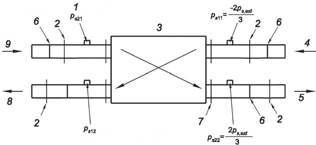
1 — измерение давления; 2 — измерение температуры и влажности; 3 — испытуемый агрегат; 4 — вытяжной воздух; 5 — приточный воздух; 6 — перфорированная пластина; 7 — соединение; 8 — удаляемый воздух; 9 — наружный воздух
