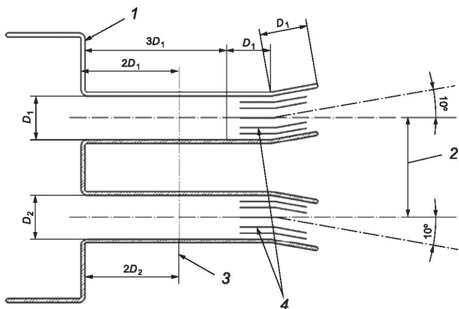
1 — стенка корпуса; 2 — расстояние между центрами воздуховодов; 3 — сечение для измерения входного давления; 4 — лопастной отвод, размещенный в воздуховоде и соединяющий измерительную камеру с корпусом
