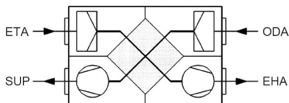
Рисунок Е.1 — Пример вентиляционного агрегата с теплообменником удаляемого/приточного воздуха
