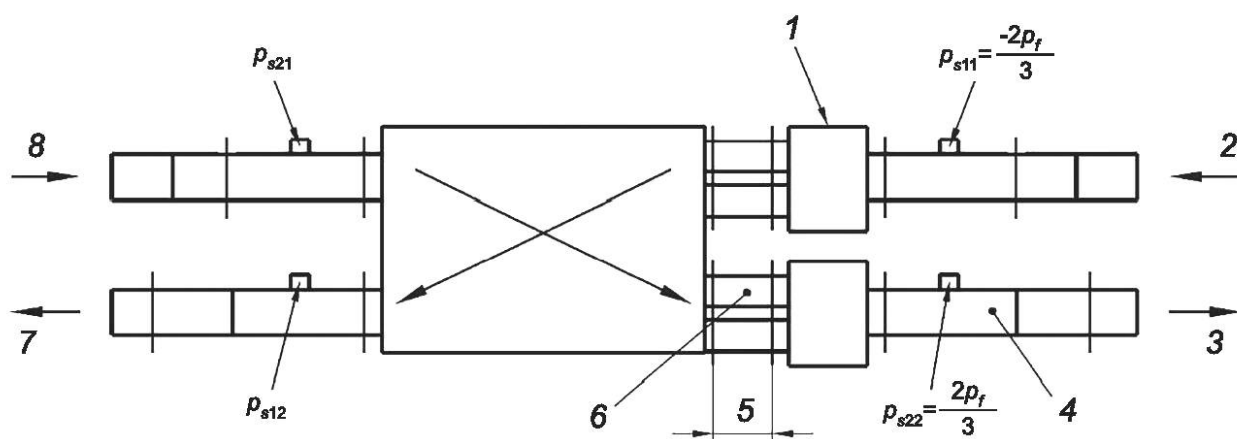
1 — соединительный короб; 2 — вытяжной воздух; 3 — приточный воздух; 4 — диаметр измерительного воздуховода D , при этом v \leq 2 м/с; 5 — расстояние от 1 до 2 D_{p2} ; 6 — диаметр патрубка D_{p2} ; 7 — удаляемый воздух; 8 — наружный воздух
