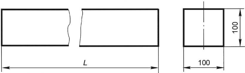
Рисунок 3 — Брус прямой, исполнение А
