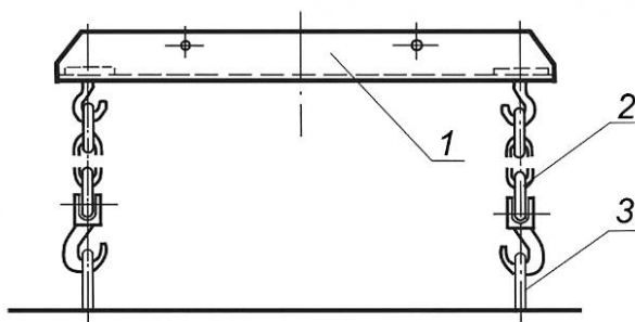
1 — балка; 2 — проставка — тип 2 (вертлюг, цепная вставка и крюк); 3 — обух
