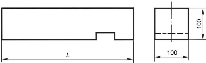
Рисунок 4 — Брус прямой, исполнение Б
