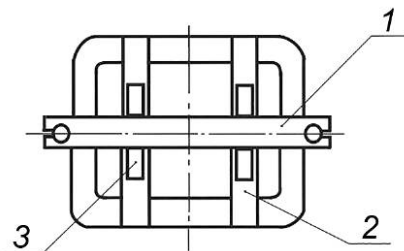
1 — балка с проставками; 2 — брус; 3 — клин
