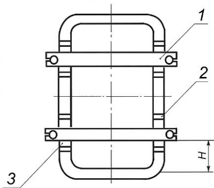
1 — балка с проставками; 2 — брус прямой; 3 — клин
