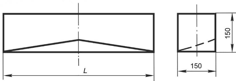
Рисунок 5 — Брус фасонный, исполнение А
