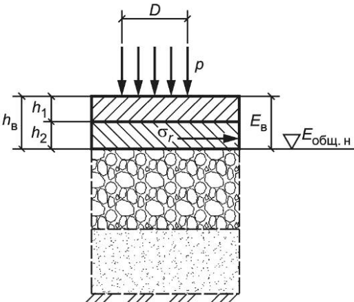
h_b — верхний слой расчетной модели; h_1, h_2 — толщины отдельных слоев асфальтобетона; E_b — средневзвешенный модуль упругости верхнего слоя; E_{\text{общ.н}} — модуль упругости упругого полупространства, ниже пакета слоев из асфальтобетона, не ограниченного снизу (нижнего слоя)
