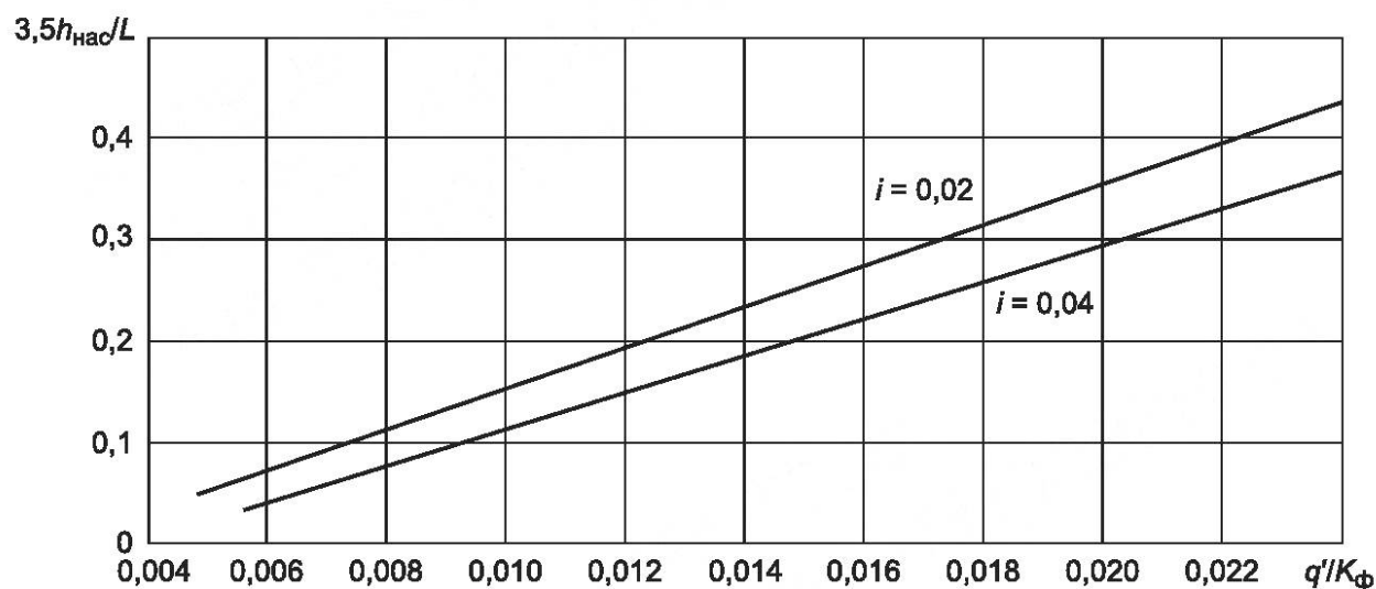
i — поперечный уклон низа дренающего слоя; L — длина пути фильтрации; q' — погонный приток воды; K_ф — коэффициент фильтрации песка, м/сут
