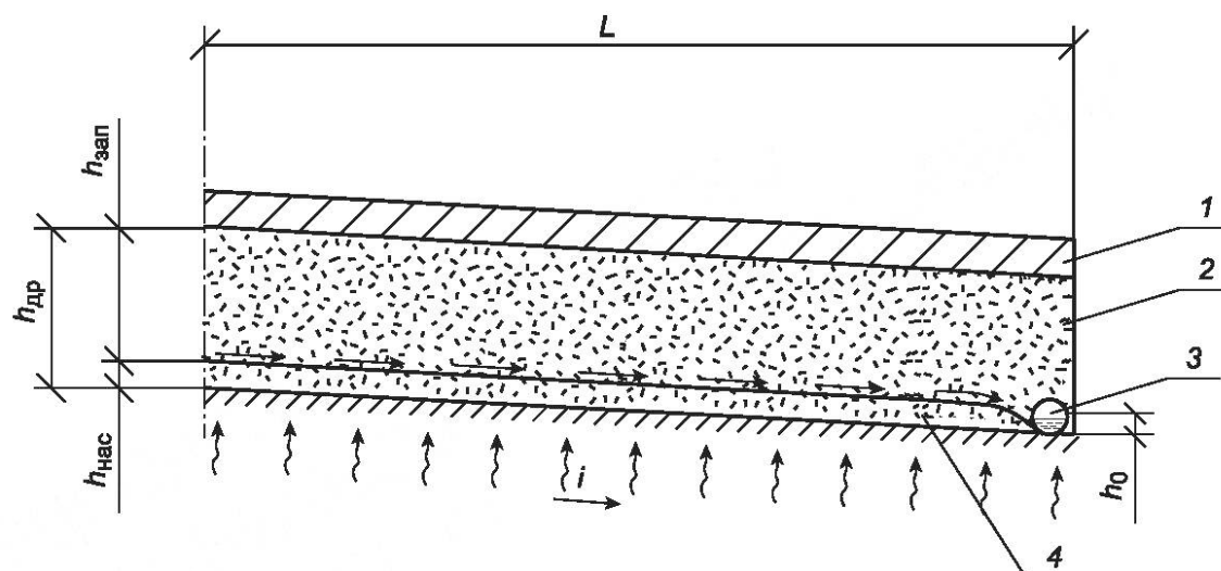
1 — слой покрытия; 2 — дренарующий слой; 3 — труба-дрена; 4 — кривая депрессии; L — длина пути фильтрации; h_{др} — толщина дренающего слоя; h_{нас} — толщина слоя, насыщенного водой; h_{зап} — толщина слоя с капиллярно-связанной водой; h_0 — уровень воды в трубе-дрене
