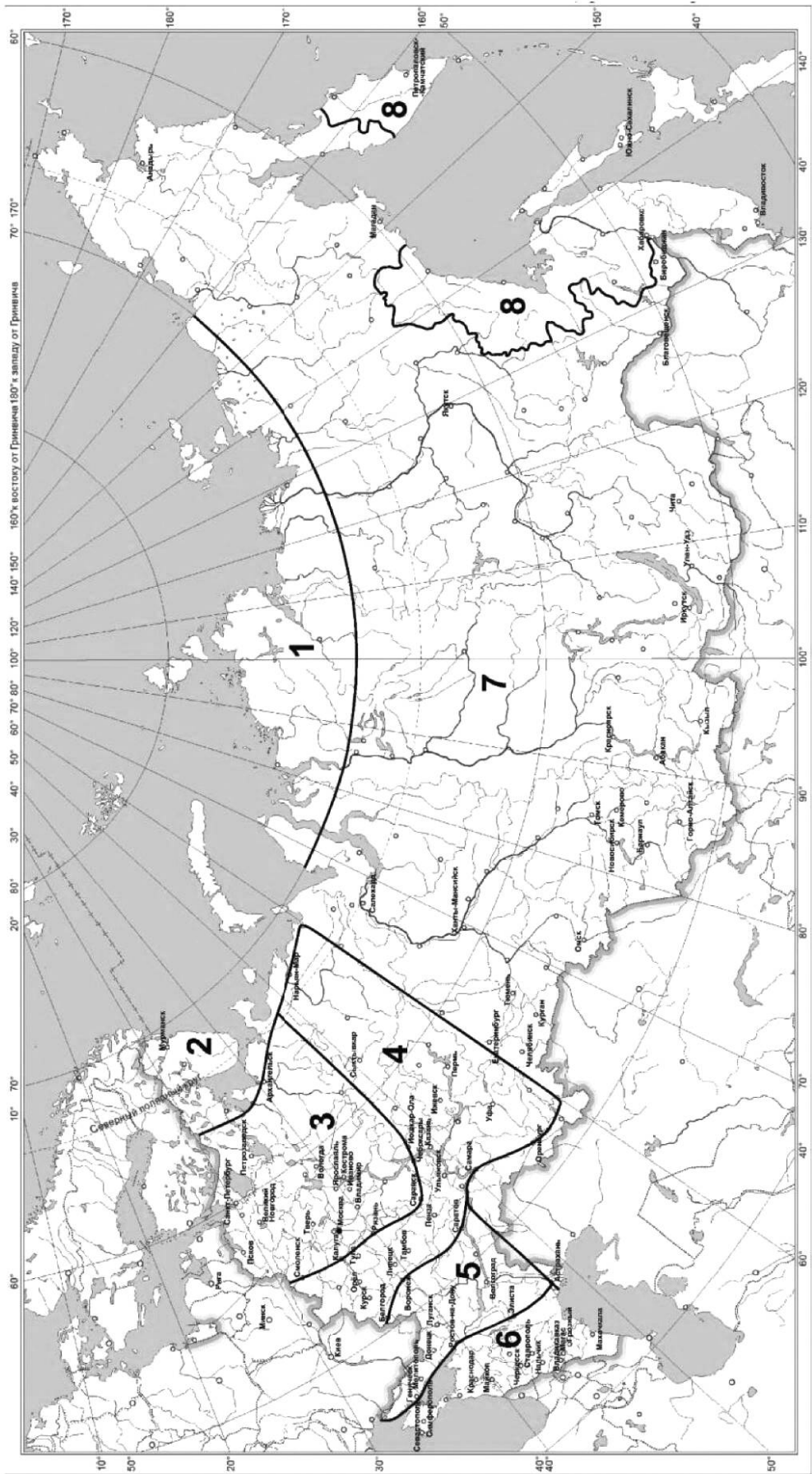
Рисунок 1 — Карта районирования по количеству расчетных дней в году T_{рад}
