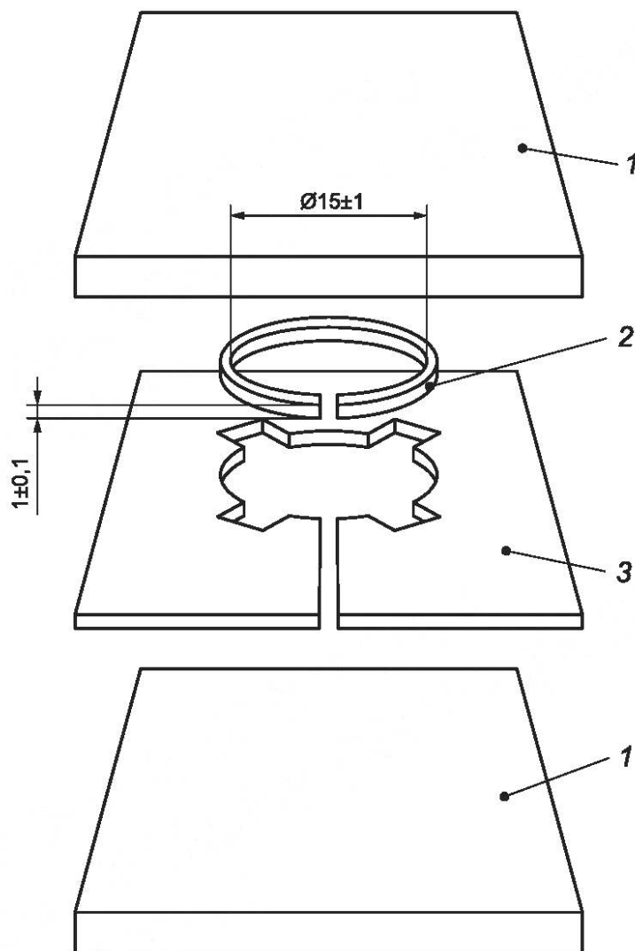
Рисунок 1 — Форма для изготовления испытываемых образцов для определения глубины отверждения, чистоты поверхности, водопоглощения, растворимости, соответствия цвета и цветостойкости
