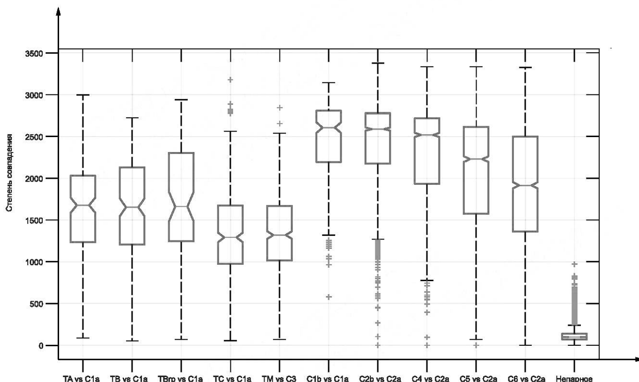
Рисунок 3 — Пример «диаграммы размаха»
