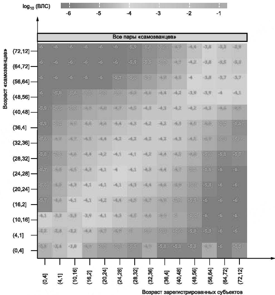
Рисунок 9 — Пример тепловой карты: изменение ВЛС из-за разницы в возрасте «самозванцев» и зарегистрированных пользователей
