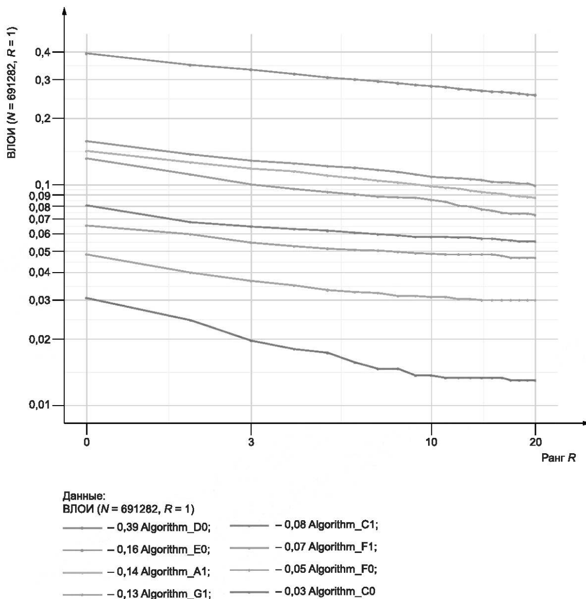
Рисунок 7 — Пример графика «ВЛОИ по рангу»
