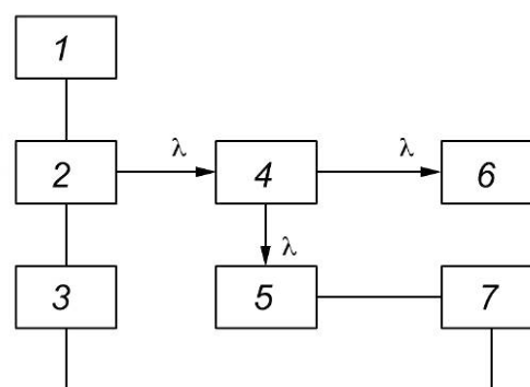
Рисунок 1 — Схема расположения средств измерений и вспомогательных устройств при измерении средней мощности импульса выходного полезного излучения
