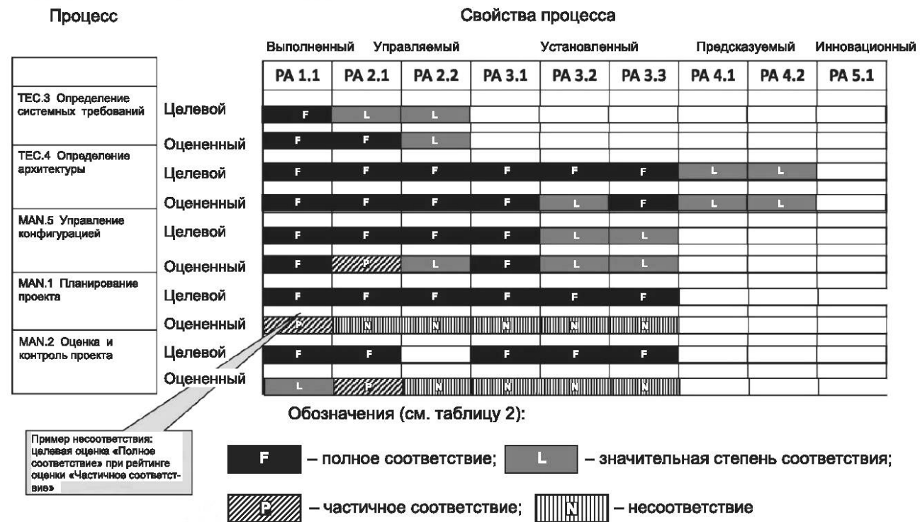
Рисунок 3 — Целевые и оцененные профили процессов
