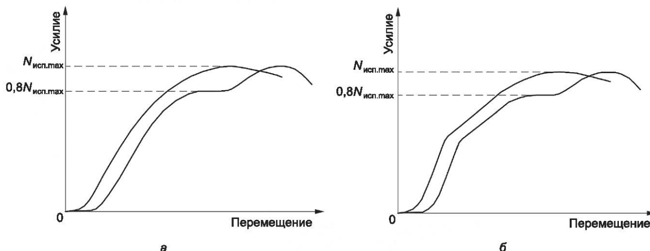
Рисунок 2 — Кривые нормального разрушения анкерного крепления без перегиба (а) и с перегибом (б) в интервале до 0,8N_{исп.мах}
