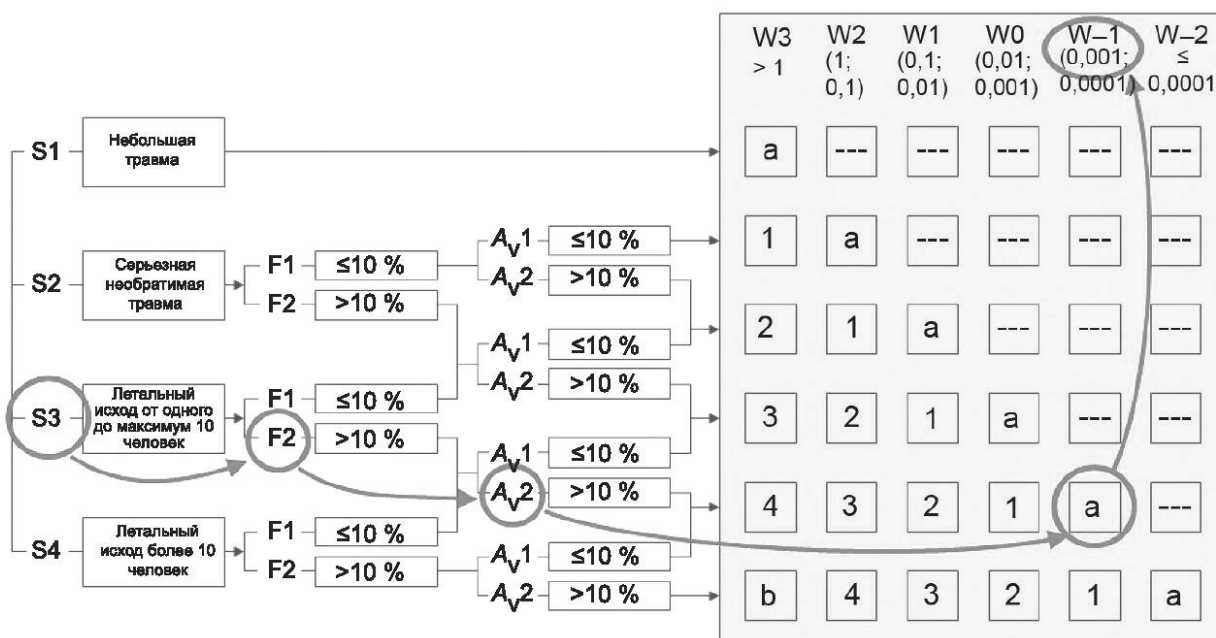
b) Рисунок 8 из VDMA 4315-1:2013-02. Турбомашины и генераторы 1)
