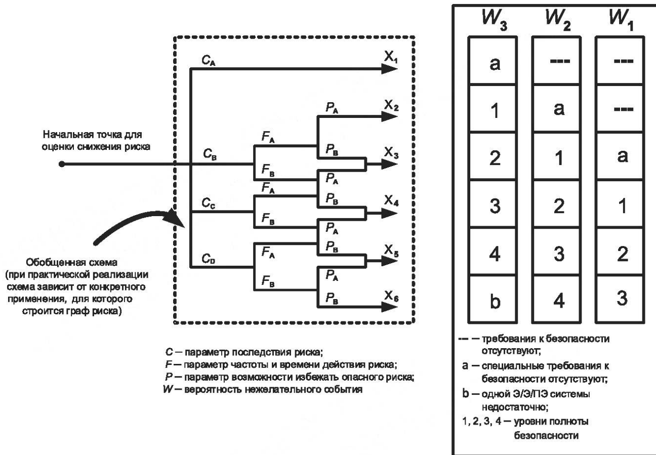
Рисунок А.7 — Граф риска для режима работы с низкой частотой запросов
