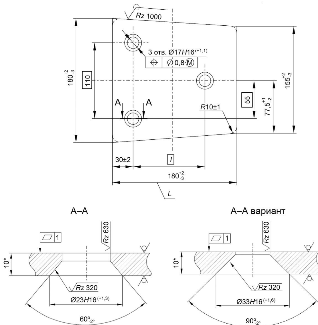
Рисунок 2 — Планка против истирания
