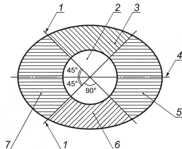
1 — взаимно перпендикулярные плоскости; 2 — купольная зона; 3 — боковая зона правая; 4 — продольная плоскость симметрии БШ; 5 — тыльная зона; 6 — боковая зона левая; 7 — лобовая зона
