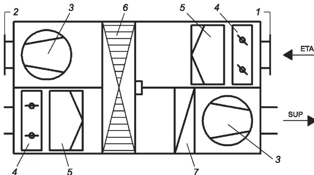
1 — пластина на входе; 2 — пластина на выходе; 3 — вентилятор; 4 — многостворчатый клапан; 5 — фильтр; 6 — рекуператор; 7 — воздушонагреватель/воздухоохладитель; ETA — вытяжной воздух; SUP — приточный воздух
