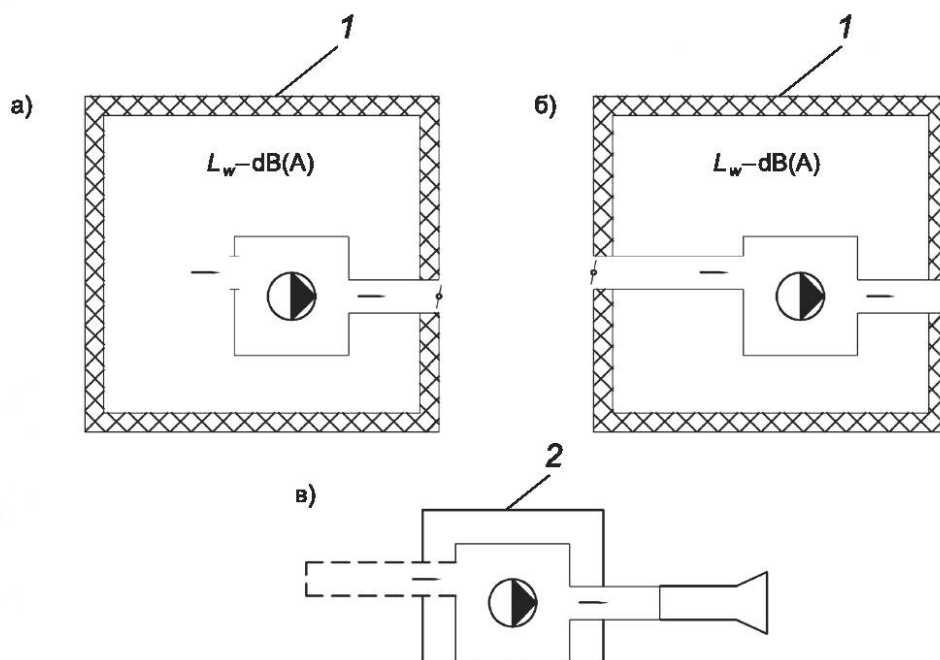
1 — реверберационная камера; 2 — измерительная поверхность
