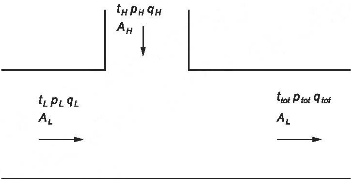
Примечание — Нижний индекс «H» относится к потоку воздуха с более высокой температурой, «L» относится к потоку воздуха с более низкой температурой, а «tot» — к потоку воздуха ниже по движению. Рисунок 11 — Параметры для расчета средней скорости и средней температуры, а также для определения коэффициента температурного перемешивания
