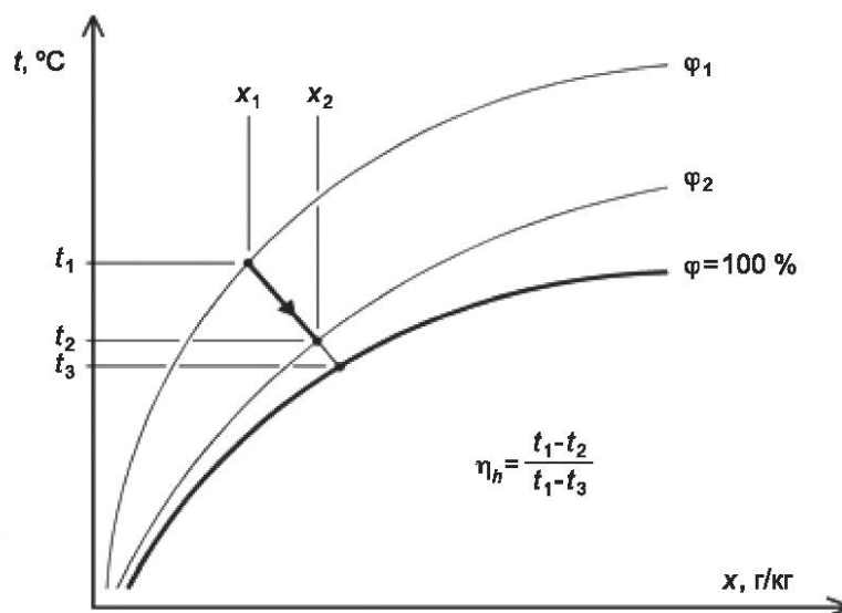
Рисунок 12 — Эффективность увлажнителя
