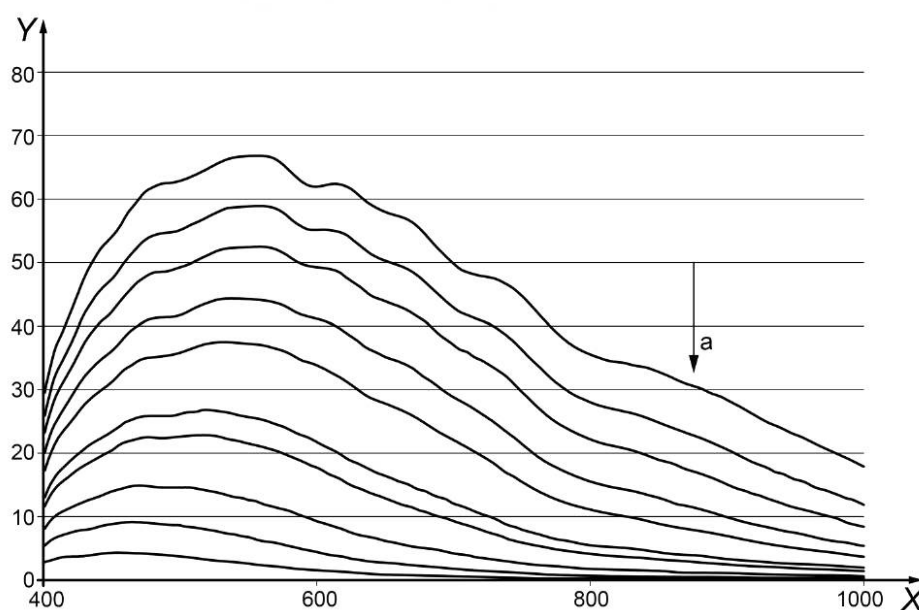
X — длина волны излучения, нм; Y — коэффициент пропускания света, %; a — направление уменьшения коэффициента пропускания света
