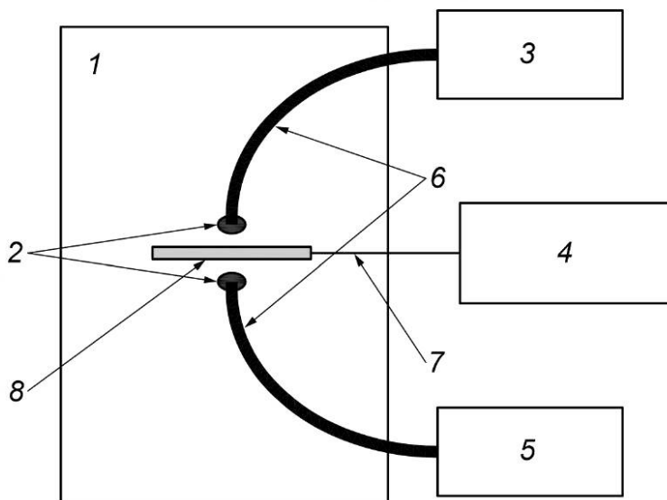
1 — термошкаф; 2 — коллимирующие линзы; 3 — источник света; 4 — блок управления переключением; 5 — спектрометр; 6 — оптические кабели; 7 — термопара с электрическими выводами; 8 — образец
