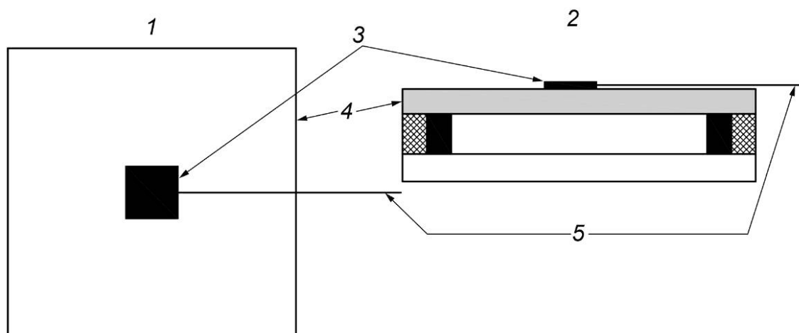
1 — образец (вид сверху); 2 — образец (вид сбоку); 3 — алюминиевая лента; 4 — поверхность образца с ЭХН; 5 — электрические выводы термопары
