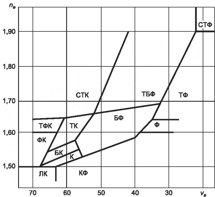
Рисунок 1 — Диаграмма «Показатель преломления n_e — коэффициент дисперсии v_e »
