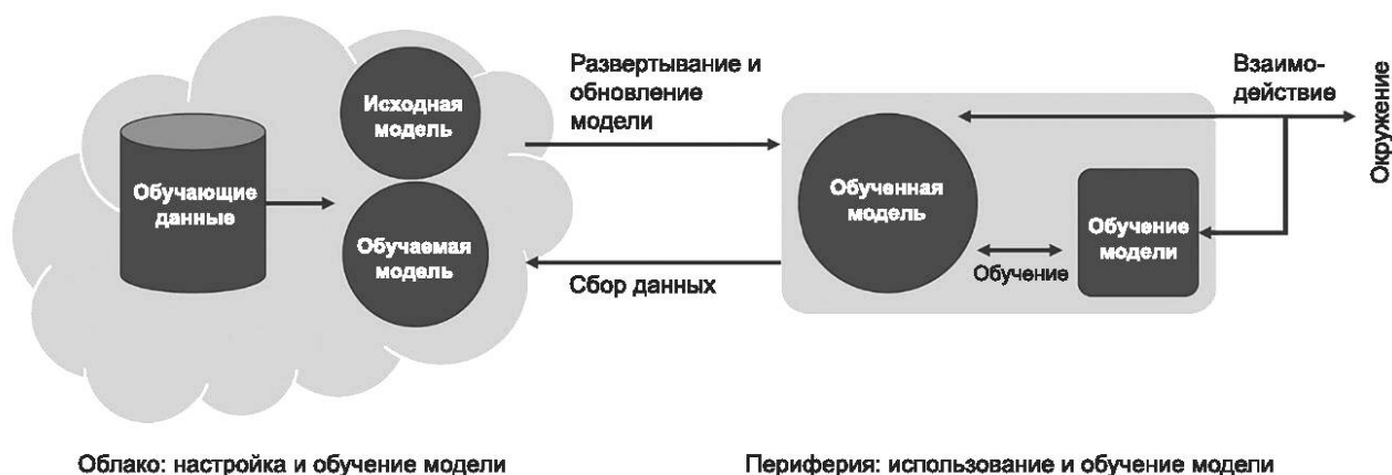
Рисунок 10 — Пример обучения модели в облаке и на периферии
