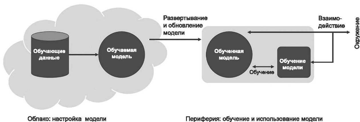
Рисунок 9 — Пример обучения модели на периферии
