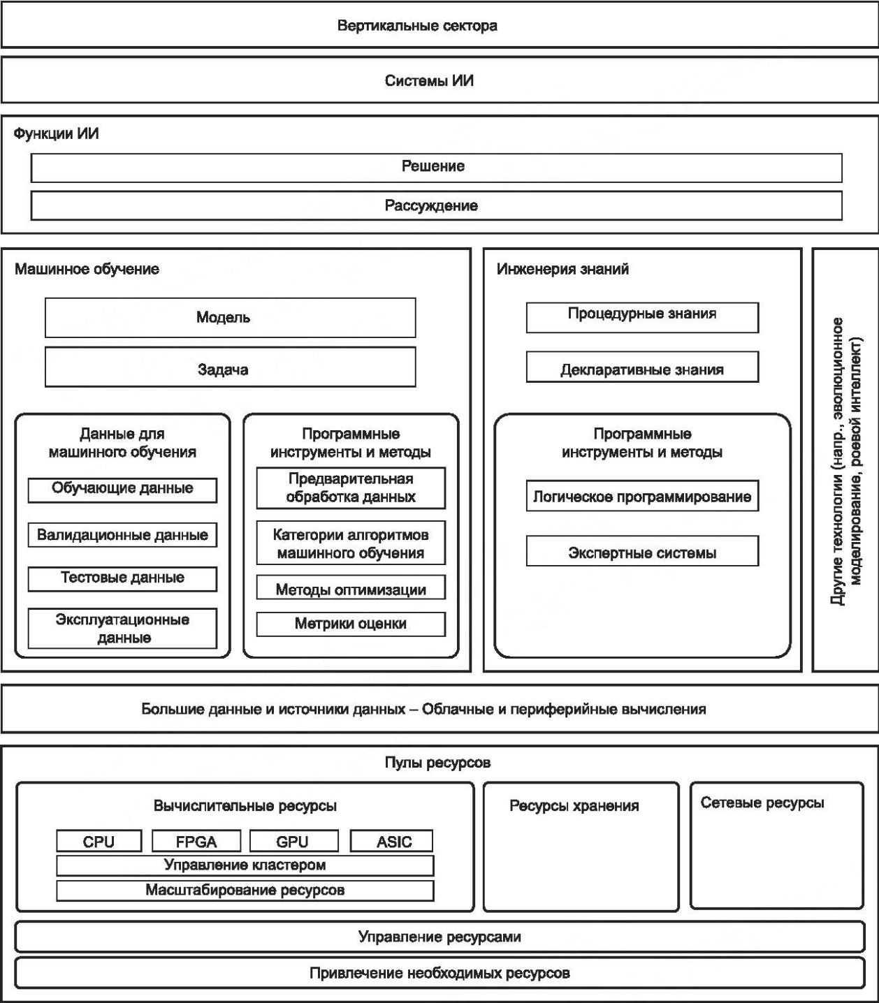
Рисунок 6 — Экосистема ИИ
