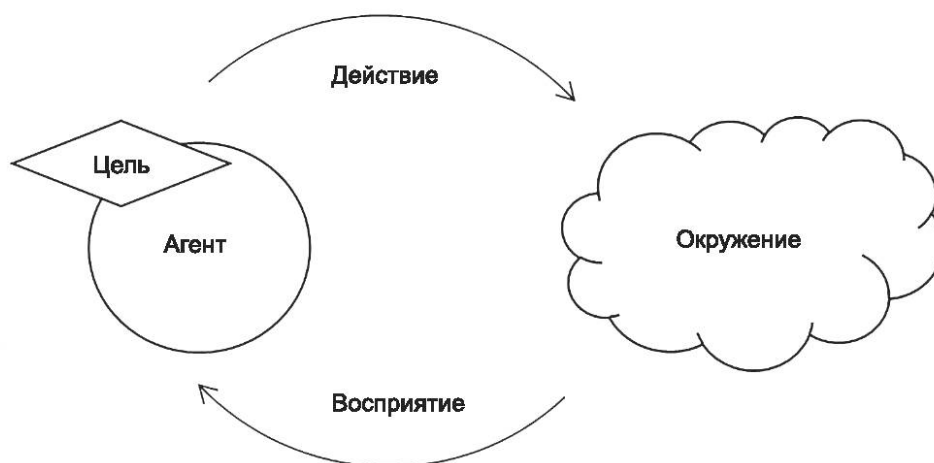
Рисунок 1 — Парадигма агента
