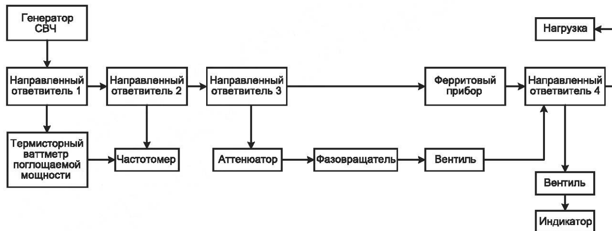
Рисунок 2 — Структурная схема установки для измерения фазового сдвига на высоком уровне мощности методом II
