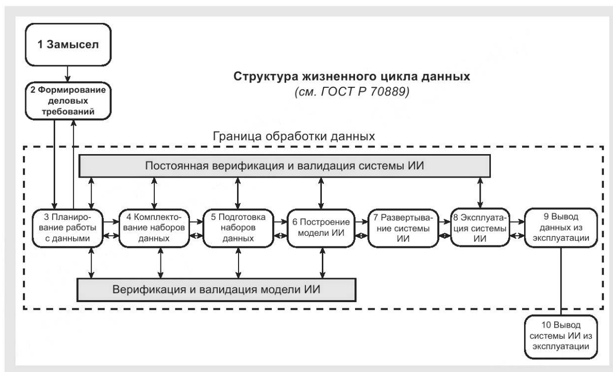
Реализация модели жизненного цикла данных для стандартов серии ГОСТ Р 71484
