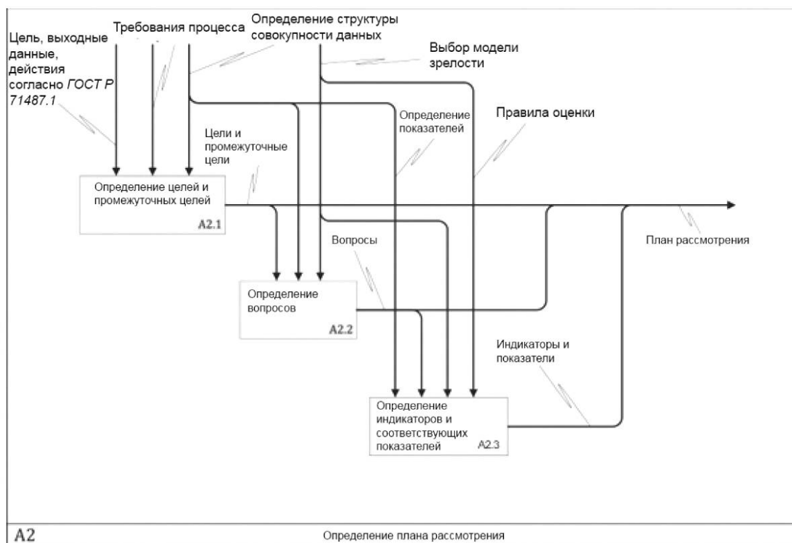
Рисунок 10 — Определение плана рассмотрения (схема модели действий A2)
