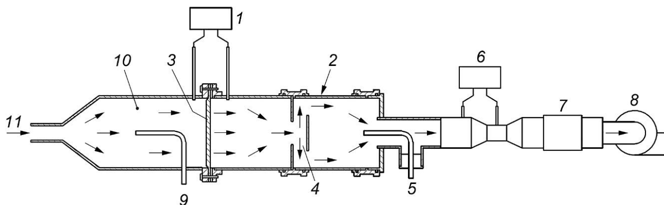
1 — манометр; 2 — испытательный канал; 3 — образец фильтрующего материала; 4 — смесительная секция; 5 — проботборная трубка после фильтра; 6 — расходомер; 7 — устройство контроля расхода воздуха; 8 — вентилятор; 9 — проботборная трубка до фильтра; 10 — канал до фильтра; 11 — контрольный аэрозоль
