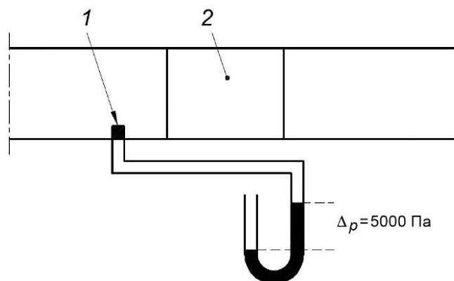
1 — заглушенное отверстие для измерения давления; 2 — секция испытательного устройства
