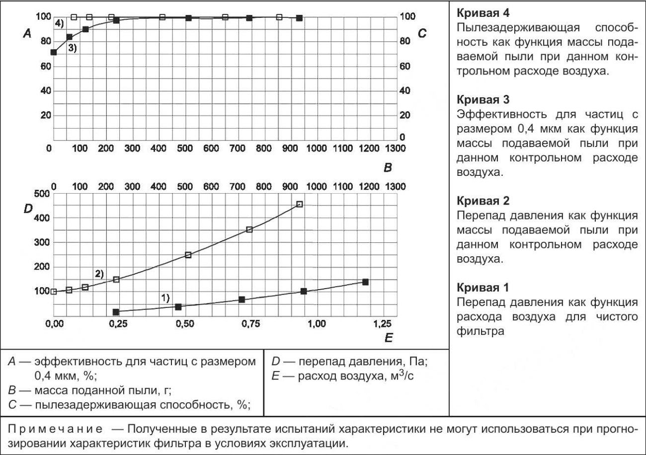
Рисунок Г.1 — Краткое представление результатов испытаний
