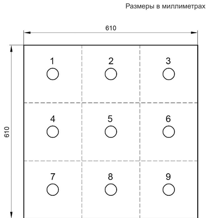
Рисунок 8 — Точки для отбора проб и измерения распределения скорости воздуха и дисперсности аэрозоля
