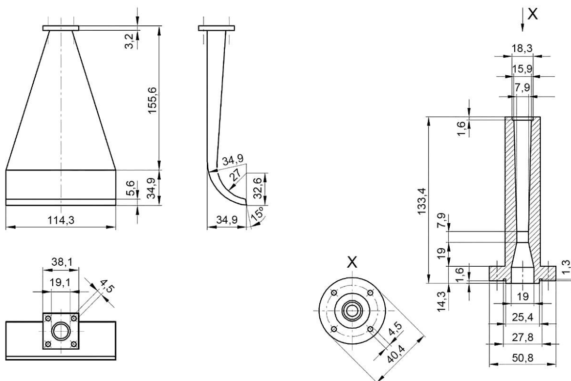
а) Пылеотборная труба
