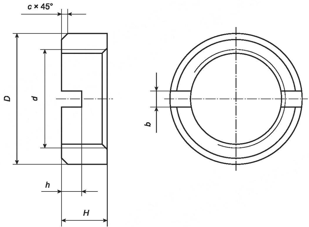
Рисунок 1 — Конструкция круглых низких гаек со шлицем
