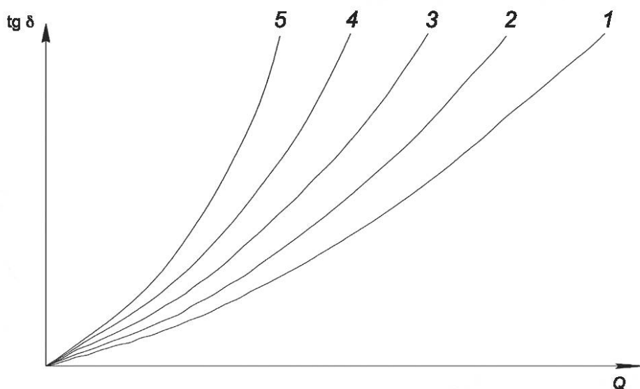
Рисунок 3 — Зависимость тангенса угла диэлектрических потерь индикатора \text{tg } \delta от количества поглощенной им влаги при разных температурах
