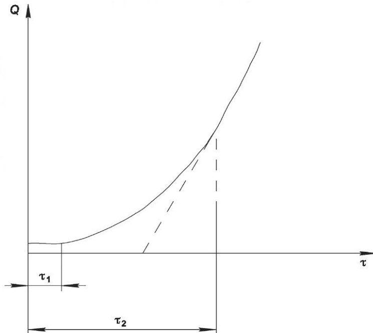
Рисунок 4 — Зависимость количества влаги Q , прошедшей через образец, от времени \tau при определении влагопроницаемости материала
