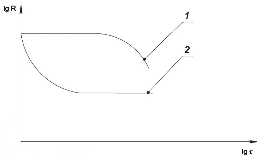
Рисунок 5 — Зависимость сопротивления на поверхности испытываемого образца от времени при оценке сорбционных свойств материала
