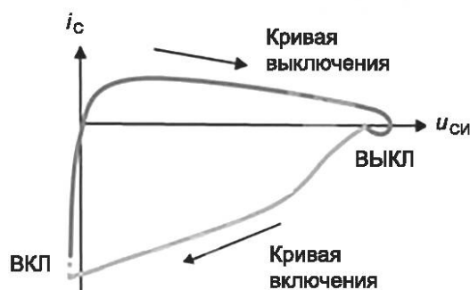
б) Переходы включения и выключения с плавной коммутацией, например, СК с низким уровнем шума в понижающем преобразователе с индуктивным запоминающим элементом
