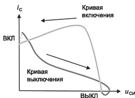
а) Включение и выключение с жестким переключением, например, высокочастотный СК в понижающем преобразователе с индуктивным запоминающим элементом
