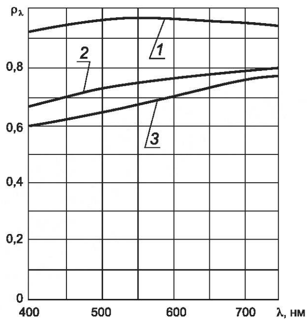
Рисунок А.1 — Кривая спектрального коэффициента диффузного отражения света \rho_\lambda полированного образца стекла марки MC20 при нормальном падении освещающего пучка света до и после облучения дозой 1 \cdot 10^5 Р
