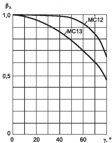
Рисунок А.2 — Индикатрисы спектральных коэффициентов яркости \beta_\lambda полированных образцов стекла марок MC12 и MC13
