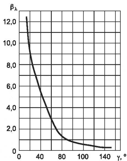
Рисунок А.5 — Индикатриса рассеяния света стекла марки МС18
