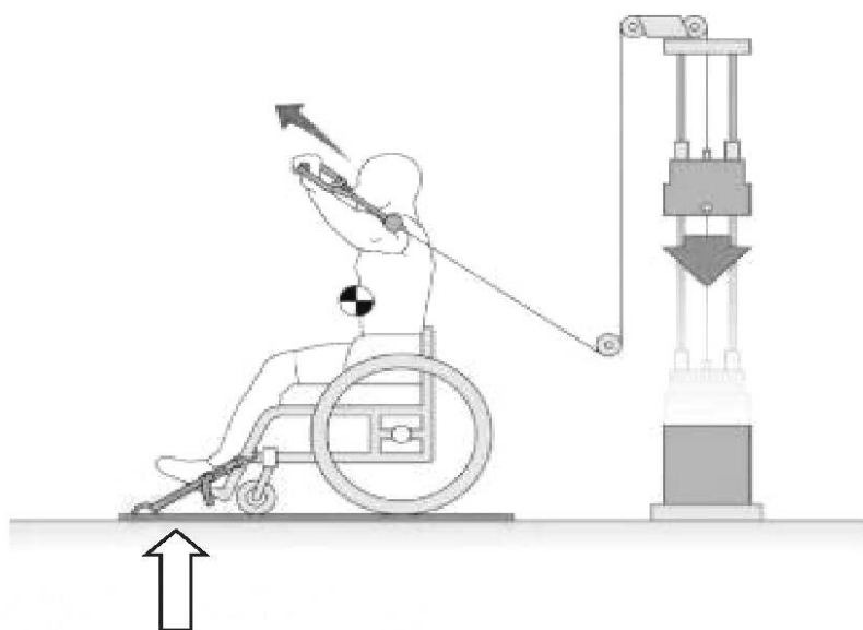
Рисунок А.2 — Пример фиксирующей тяги крепления кресла-коляски
