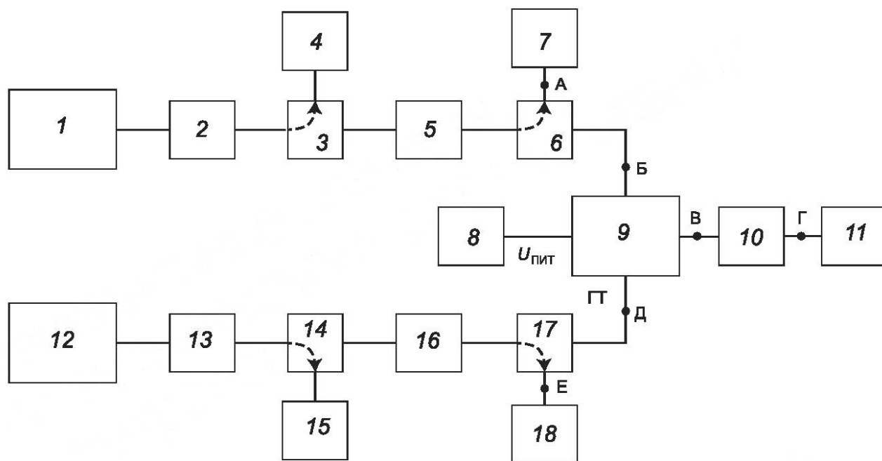
1 — ГН1; 2, 13 — изолятор 1; 3, 6, 14, 17 — направленный ответвитель; 4, 15 — измеритель частоты; 5, 16 — регулируемый аттенуатор; 7 — измеритель мощности 1; 8 — ИП; 9 — ИУ; 10 — фильтр; 11 — измеритель мощности 3; 12 — ГН2; 18 — измеритель мощности 2
