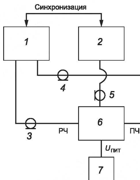
Рисунок 2 — Структурная схема измерительного стенда измерения потерь преобразования
