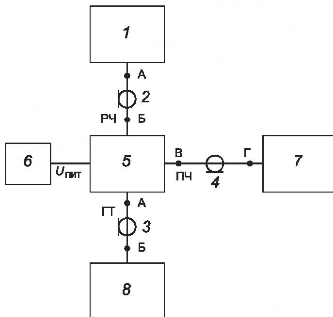
1 — ГН1; 2, 3, 4 — КС; 5 — ИУ; 6 — ИП; 7 — АС; 8 — ГН2
