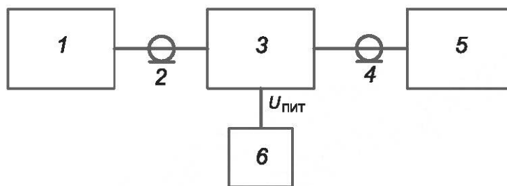
Рисунок 1 — Структурная схема измерительного стенда измерения рабочего диапазона частоты МИС
