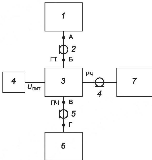
1 — ГН; 2, 4, 5 — КС; 3 — ИУ; 6 — АС; 7 — согласованная нагрузка
