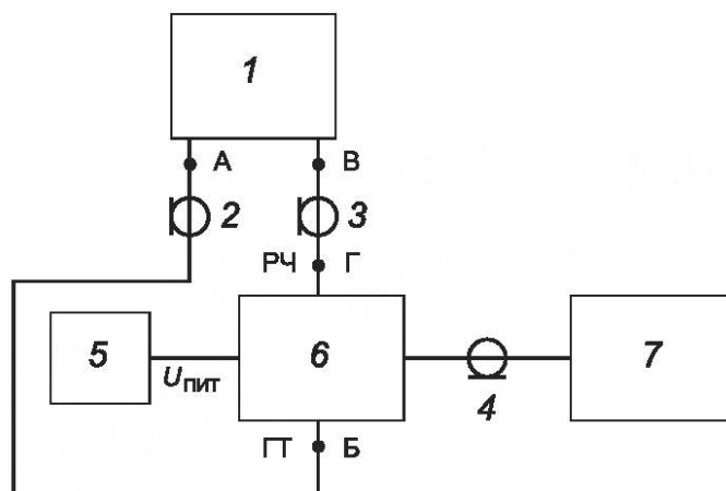
1 — ВАЦ; 2, 3, 4 — КС; 5 — ИП; 6 — ИУ; 7 — согласованная нагрузка
