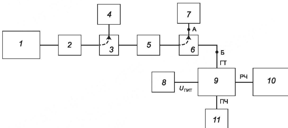
1 — ГН; 2 — изолятор; 3 — направленный ответвитель; 4 — измеритель частоты; 5 — регулируемый аттенуатор; 6 — направленный ответвитель; 7 — измеритель мощности; 8 — ИП; 9 — ИУ; 10 — АС; 11 — согласованная нагрузка
