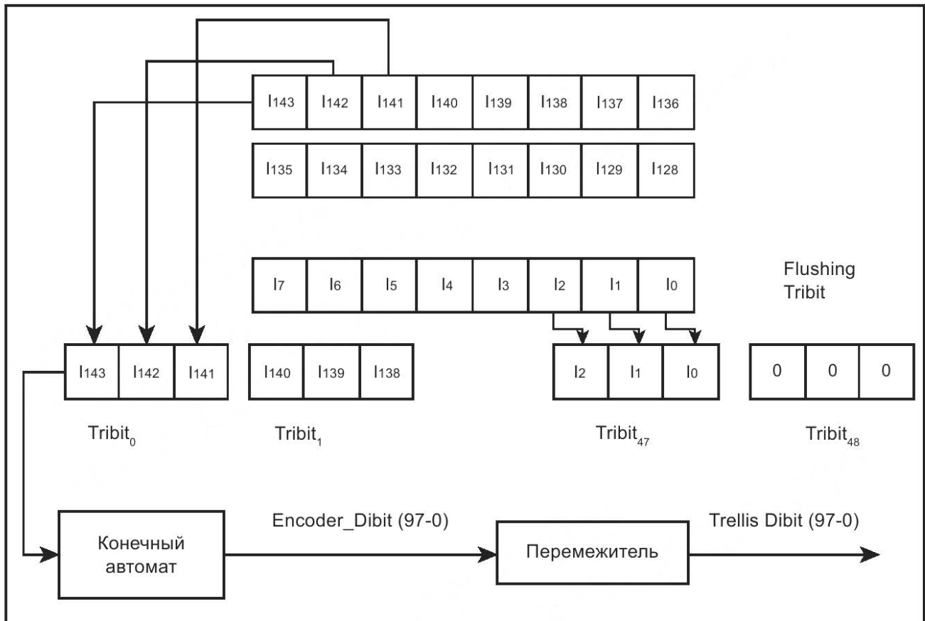
Рисунок Б.8 — Процедура кодирования треллис-кодом \frac{3}{4}
