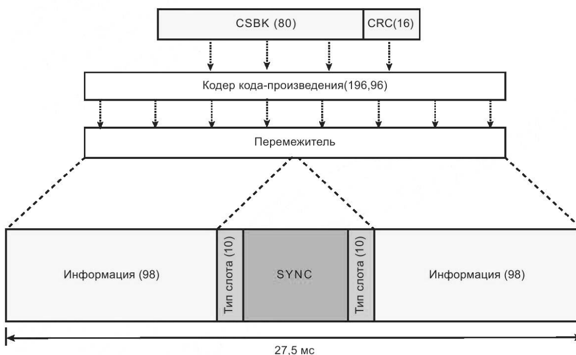
Рисунок 69 — Формирование CSBK
