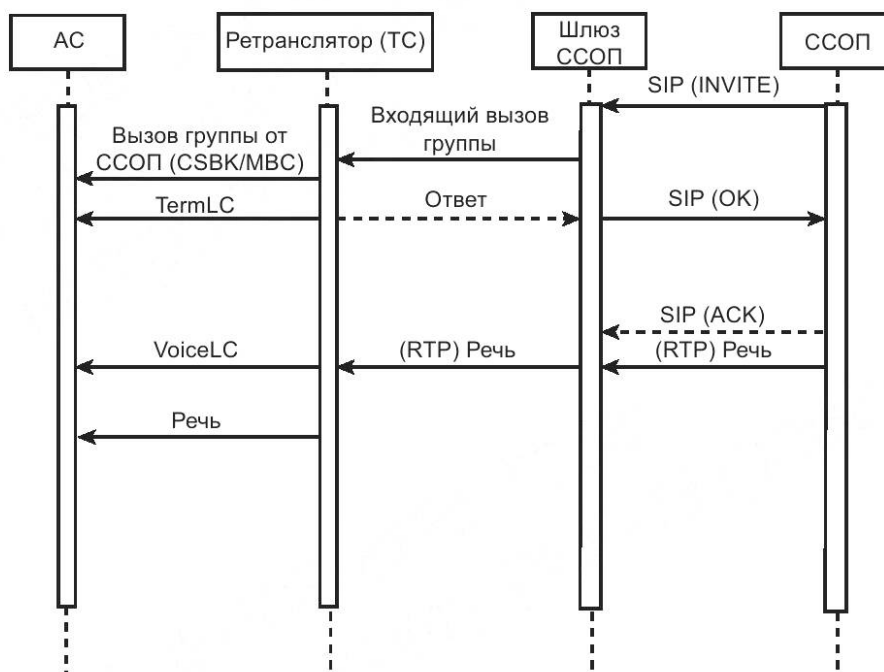
Рисунок А.6 — Последовательность установки соединения с телефонным шлюзом ССОП при групповом вызове
