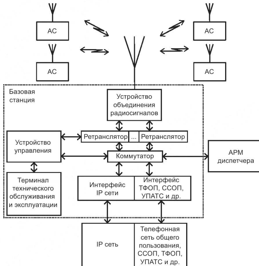
Рисунок 11 — Базовая станция
