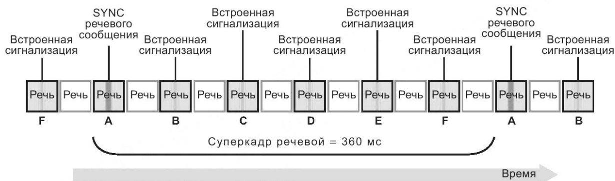
Рисунок 24 — Речевой суперкадр
