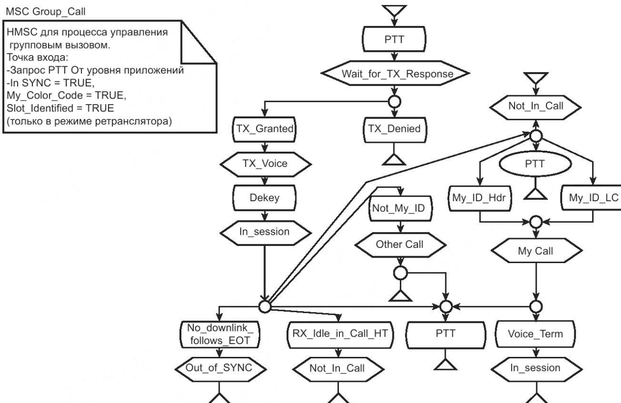
Рисунок 92 — HMSC для передачи группового вызова
