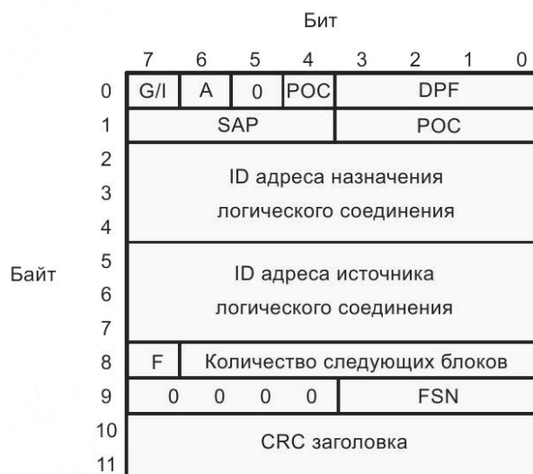
Рисунок 110 — Специальный первый блок заголовка для неподтверждаемого пакета
