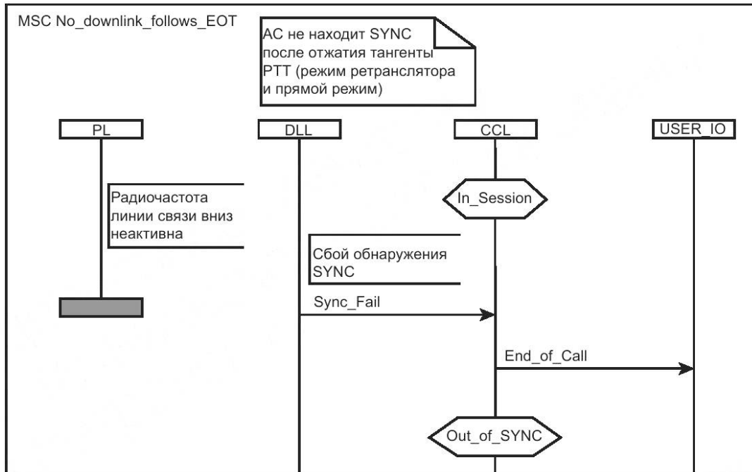
Рисунок 102 — MSC для No_Outbound_Follow_EOT
