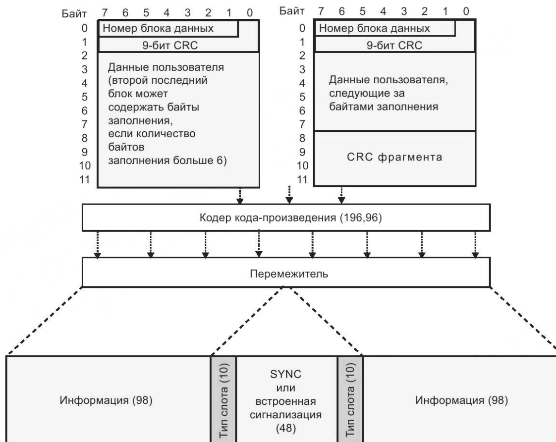
Рисунок 122 — Формат блока данных с подтверждением и FEC со скоростью кодирования \frac{1}{2}
