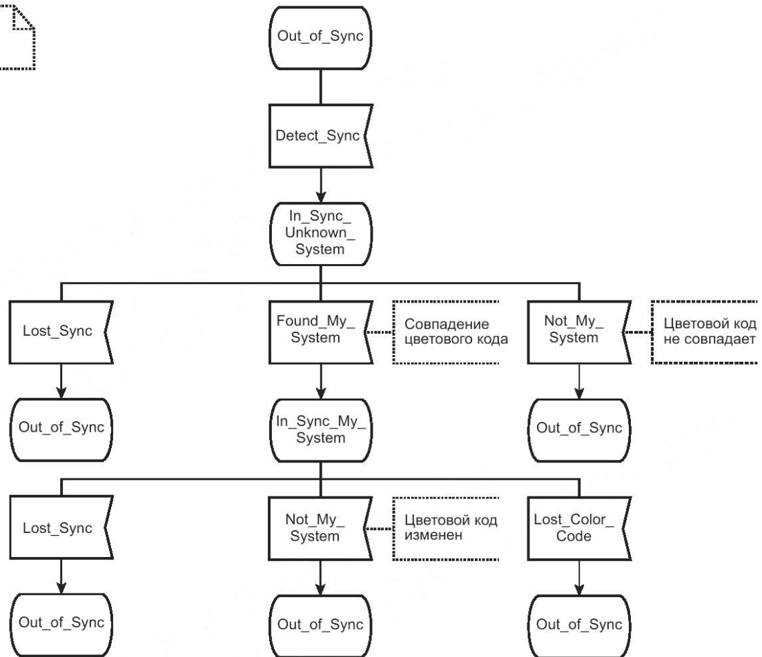
Рисунок Е.1 — SDL-диаграмма АС уровня 1, прямой режим
