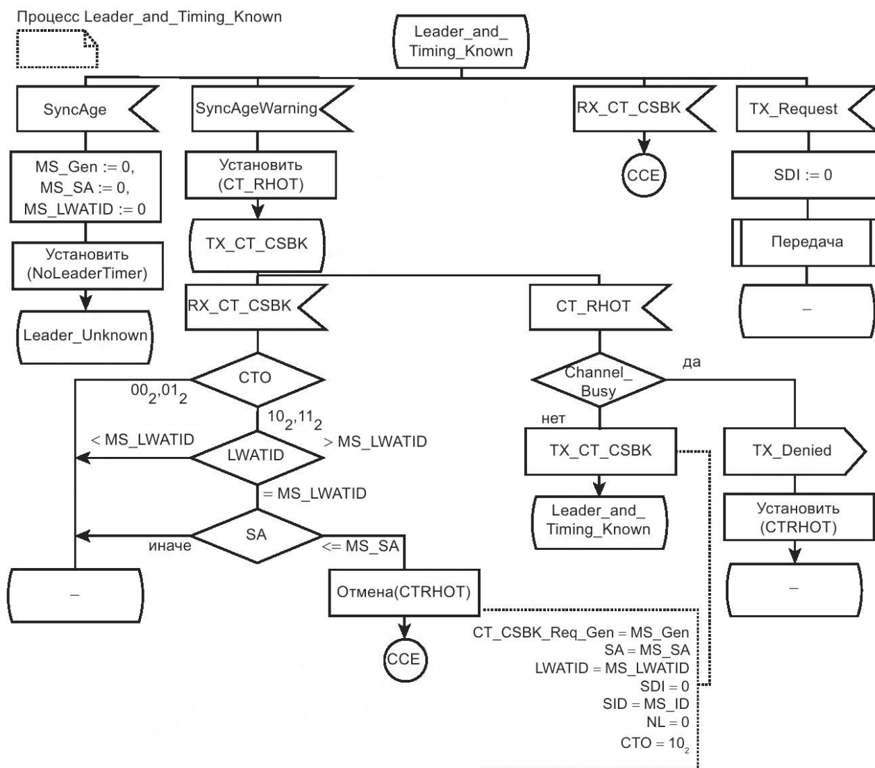
Рисунок 81 — SDL для состояния Leader_and_Timing_Known
