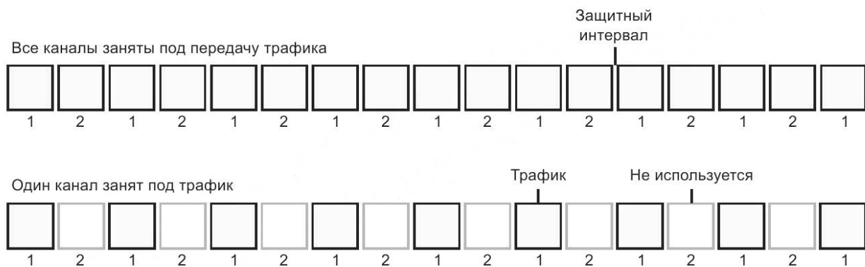
Рисунок 22 — Варианты передачи информации с помощью каналов с защитным временным интервалом
