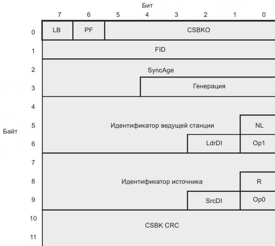
Рисунок 129 — Структура СТ_CSBK PDU
