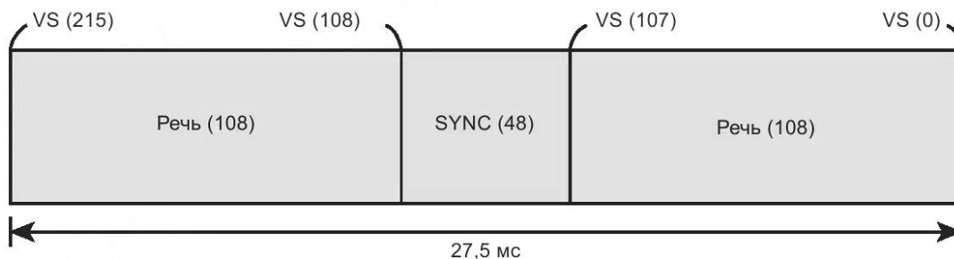
Рисунок 56 — Речевой пакет с синхронизацией
