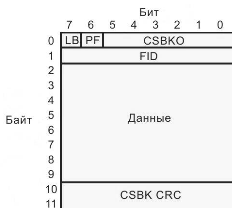
Рисунок 68 — Структура CSBK
