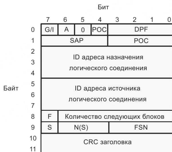
Рисунок 111 — Специальный первый блок заголовка для подтверждаемого пакета
