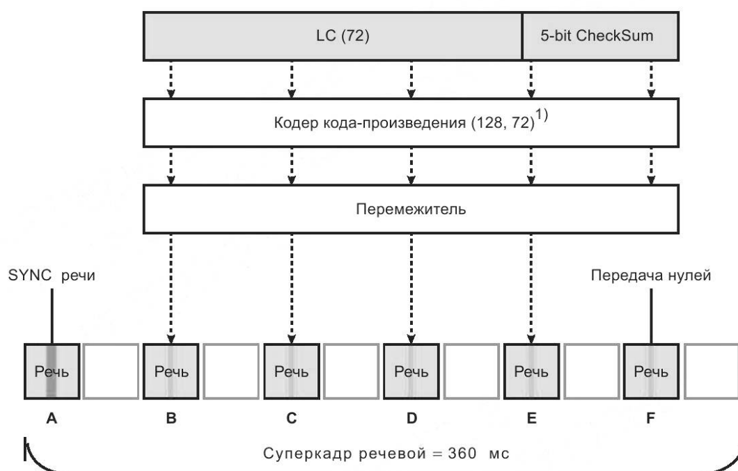
Рисунок 65 — Речевой суперкадр
