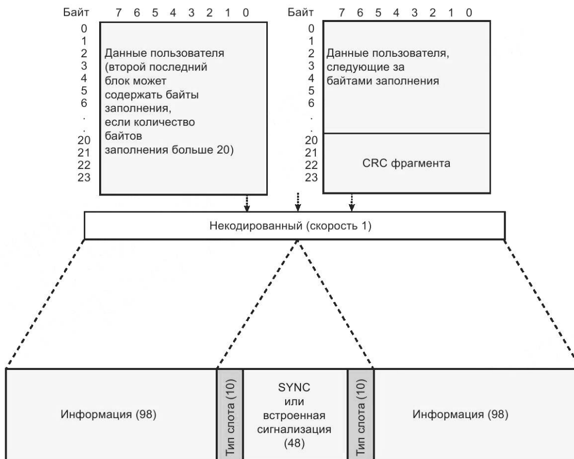
Рисунок 120 — Формат блока данных без подтверждения в режиме «без кодирования» («скорость кодирования 1»)
