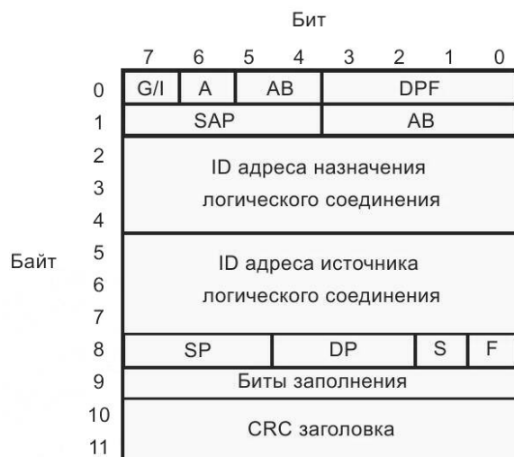
Рисунок 115 — Специальный первый блок заголовка для пакета коротких неопределенных данных
