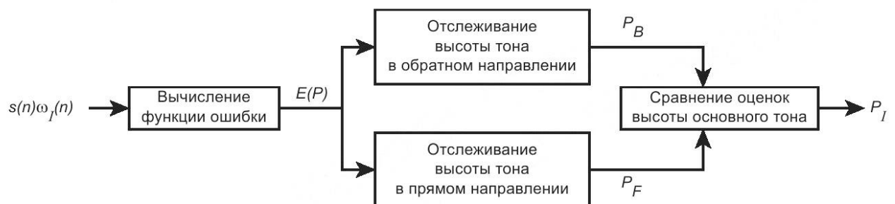
Рисунок К.4 — Первоначальная оценка высоты тона
