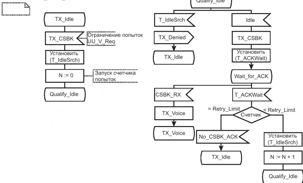
Процесс OACSU_SCBK_TX
