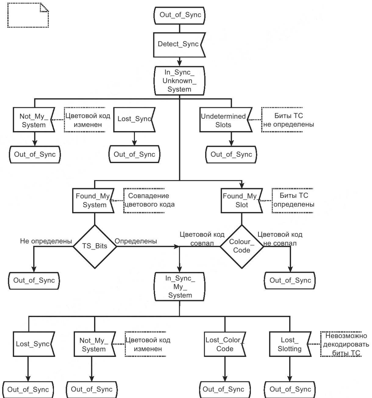
Рисунок E.2 — SDL-диаграмма AC уровня 1, режим ретранслятора
