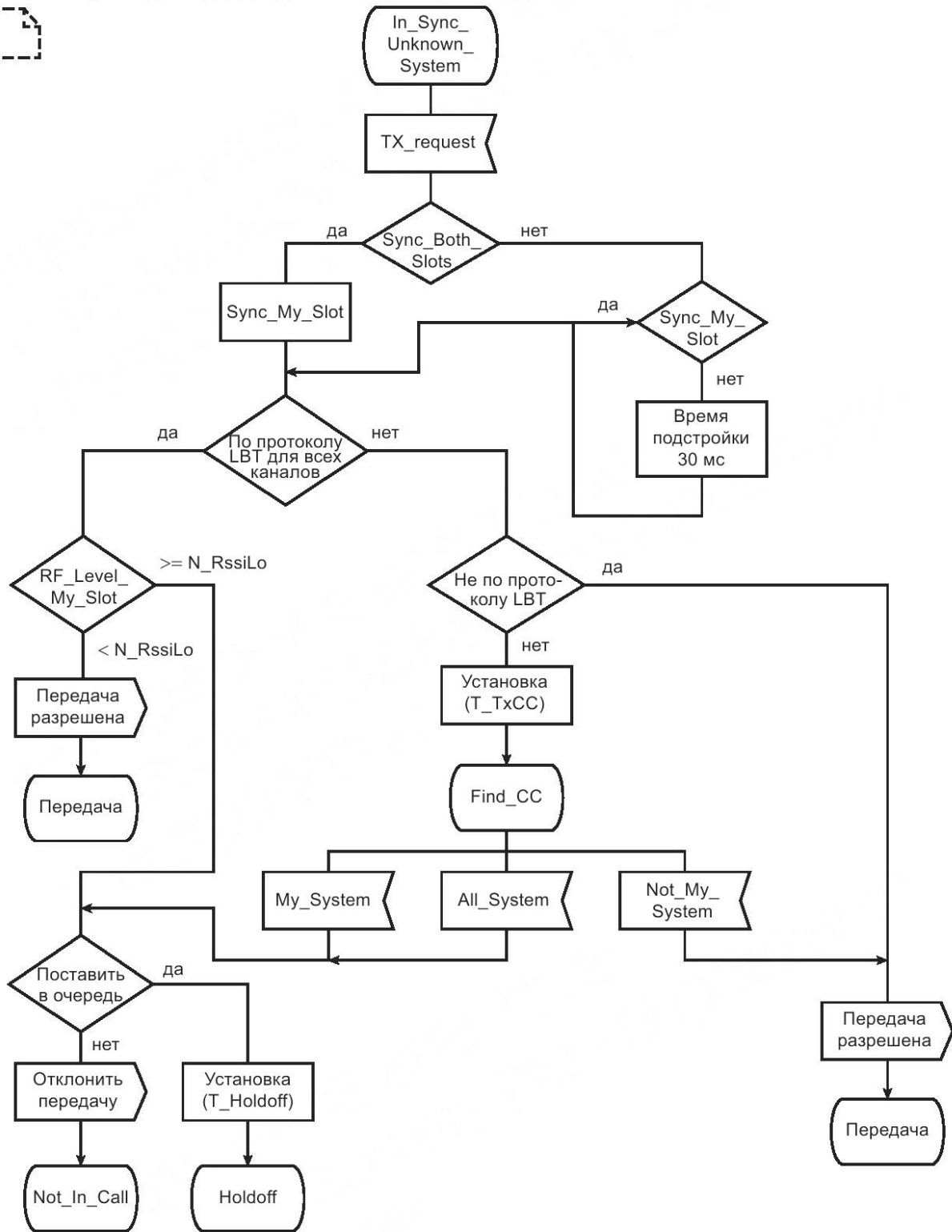
Рисунок 39 — SDL-диаграмма In_Sync_Unknown_System
