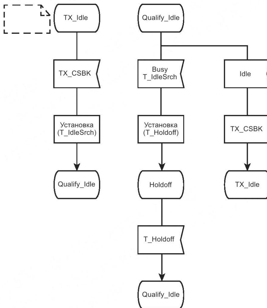
Процесс FNS_NACK_CSBK_TX
