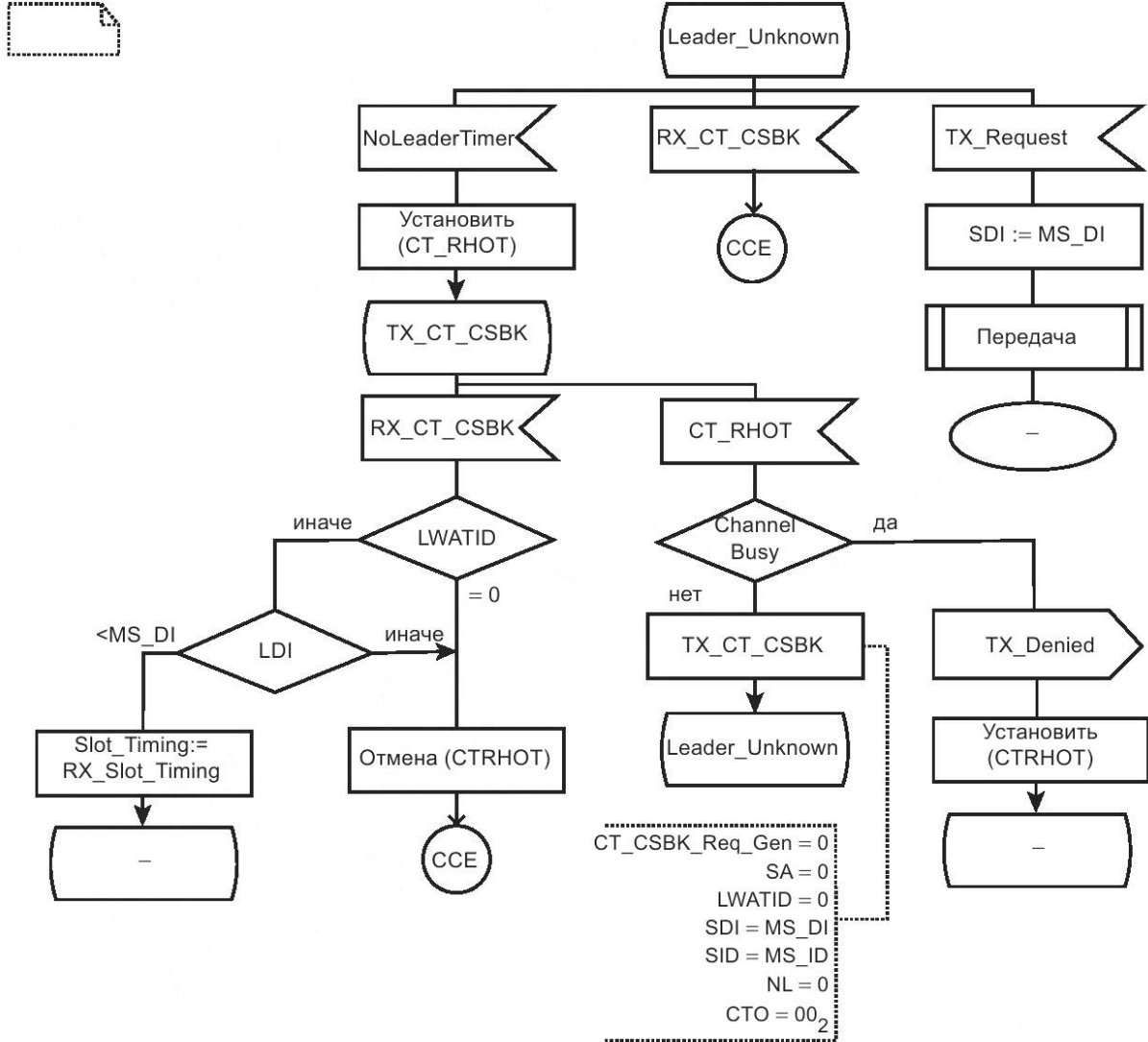
Рисунок 80 — SDL для состояния Leader_Unknown
