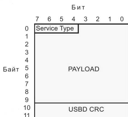
Рисунок 128 — Структура USBД
