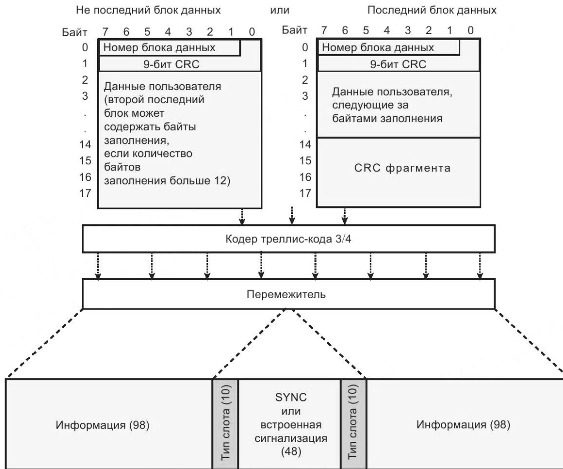
Рисунок 121 — Формат блока данных с подтверждением достоверности и треллис-кодом со скоростью кодирования \frac{3}{4}
