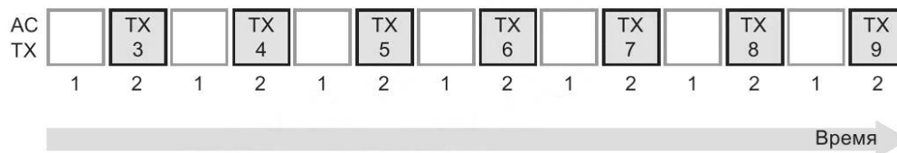
Рисунок 32 — Временная диаграмма прямого режима TDMA
