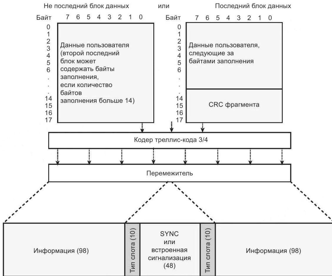
Рисунок 119 — Формат блока данных без подтверждения с FEC со скоростью кодирования \frac{3}{4}
