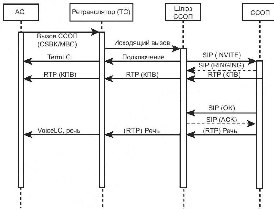
Рисунок А.2 — Последовательность установки соединения со шлюзом ССОП
