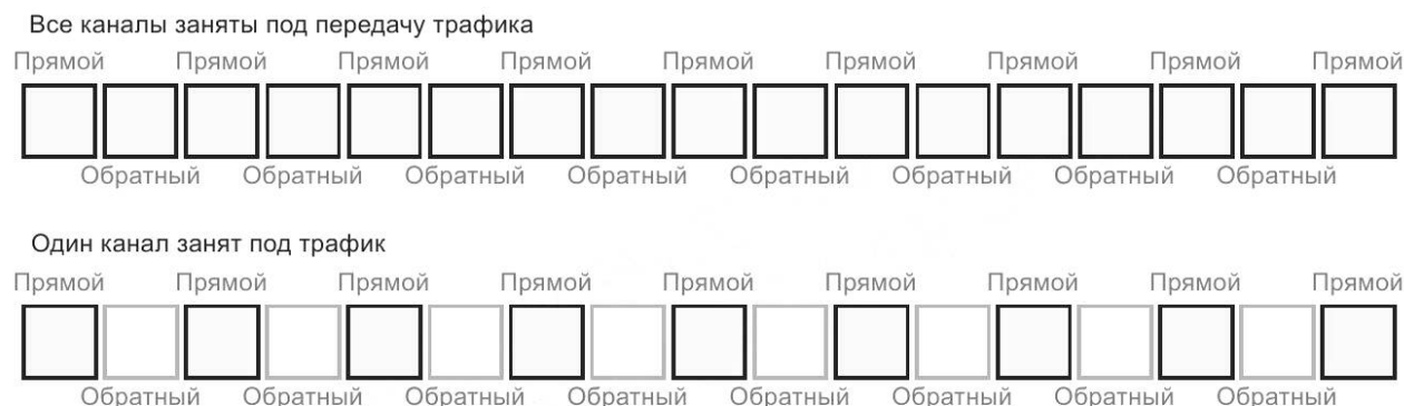
Рисунок 23 — Двухнаправленный канал
