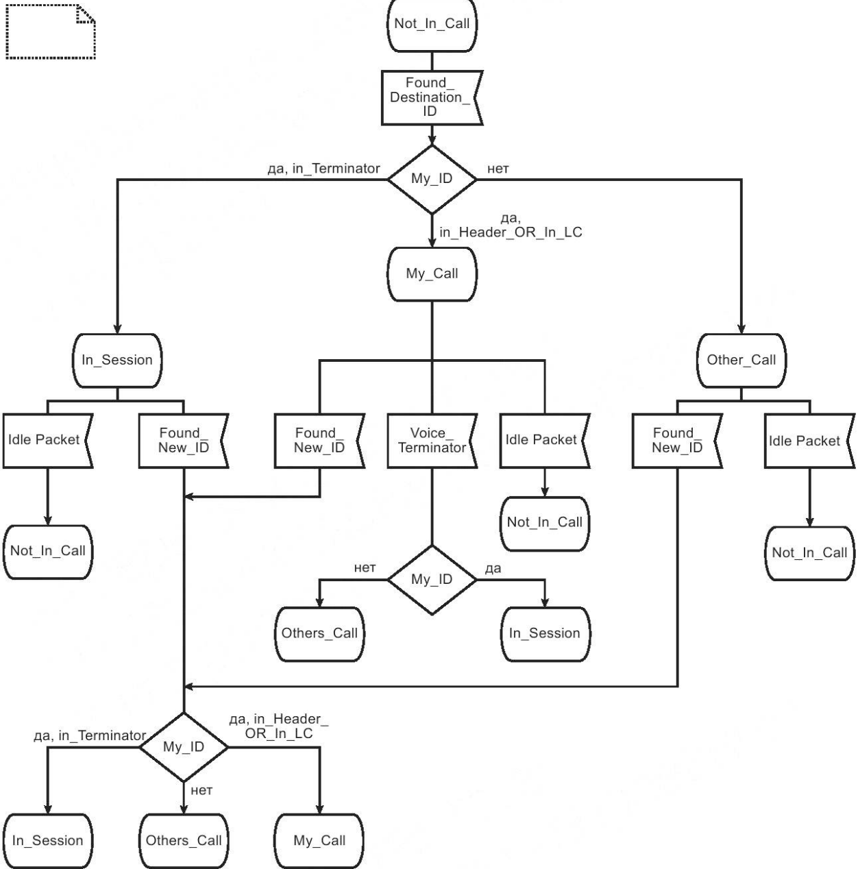
Рисунок Е.3 — SDL-диаграмма АС уровня 2
