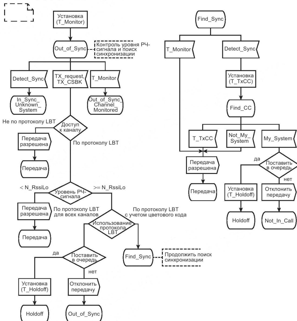
Рисунок 33 — SDL-диаграмма Out\_of\_Sync
