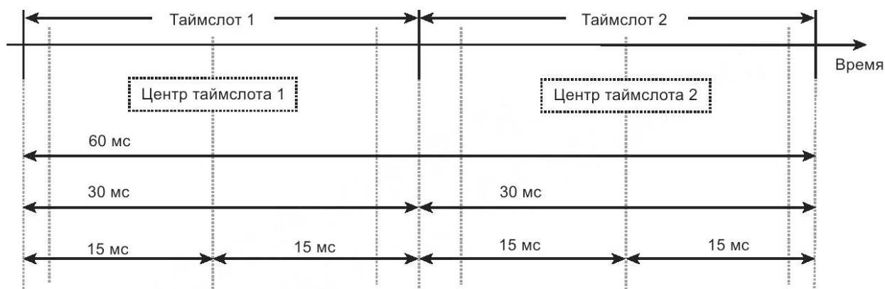
Рисунок 131 — TDMA-кадр
