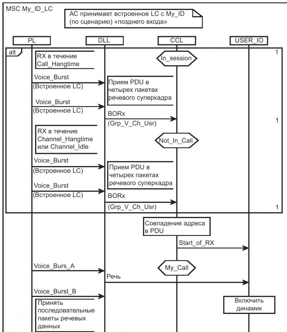
Рисунок 97 — MSC для My_ID_LC
