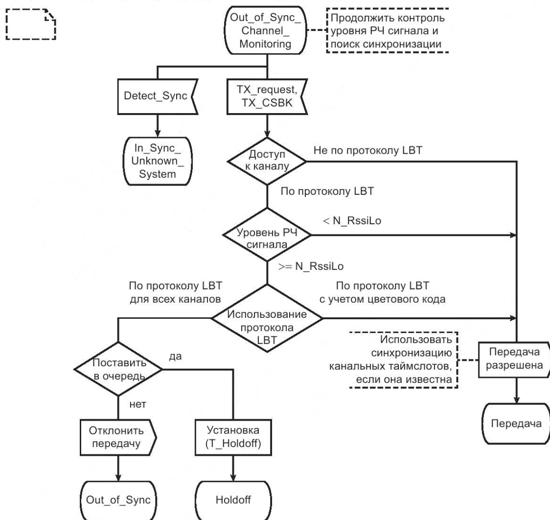
Рисунок 38 — SDL-диаграмма Out_of_Sync_Channel_Monitored
