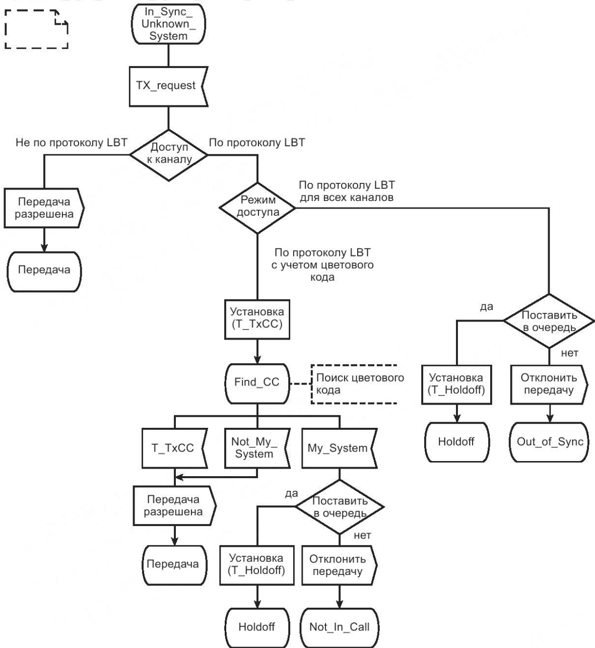
Рисунок 35 — SDL-диаграмма In_Sync_Unknown_System
