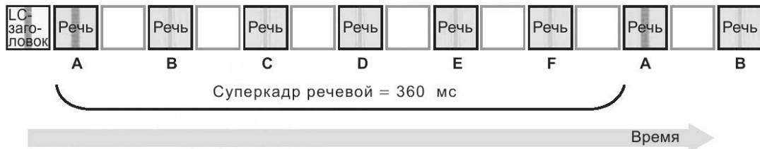
Рисунок 25 — Речевое иницирование с LC-заголовком
