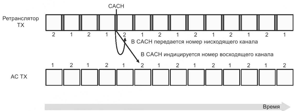
Рисунок 9 — Передача указателя о номере таймслота доступного канала
