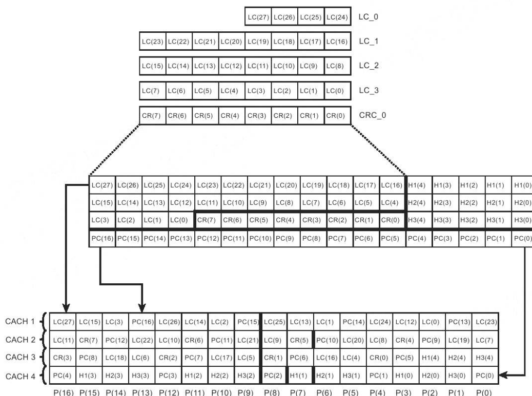
Рисунок Б.7 — Структура пакетов с CACH
