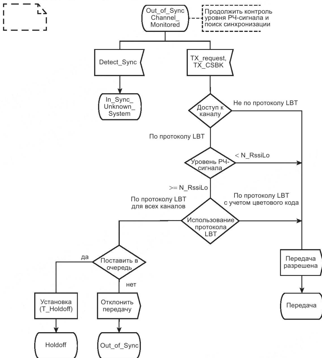
Рисунок 34 — SDL-диаграмма Out_of_Sync_Channel_Monitored
