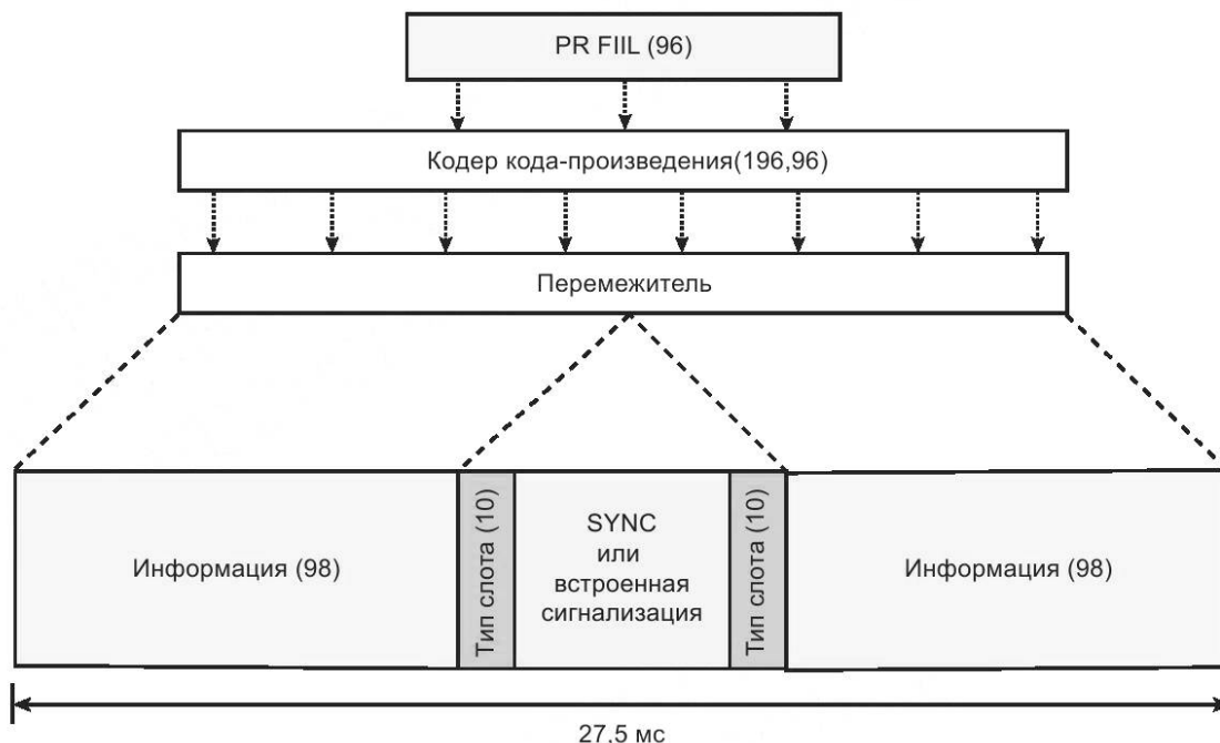
Рисунок 70 — Формирование сообщения Idle
