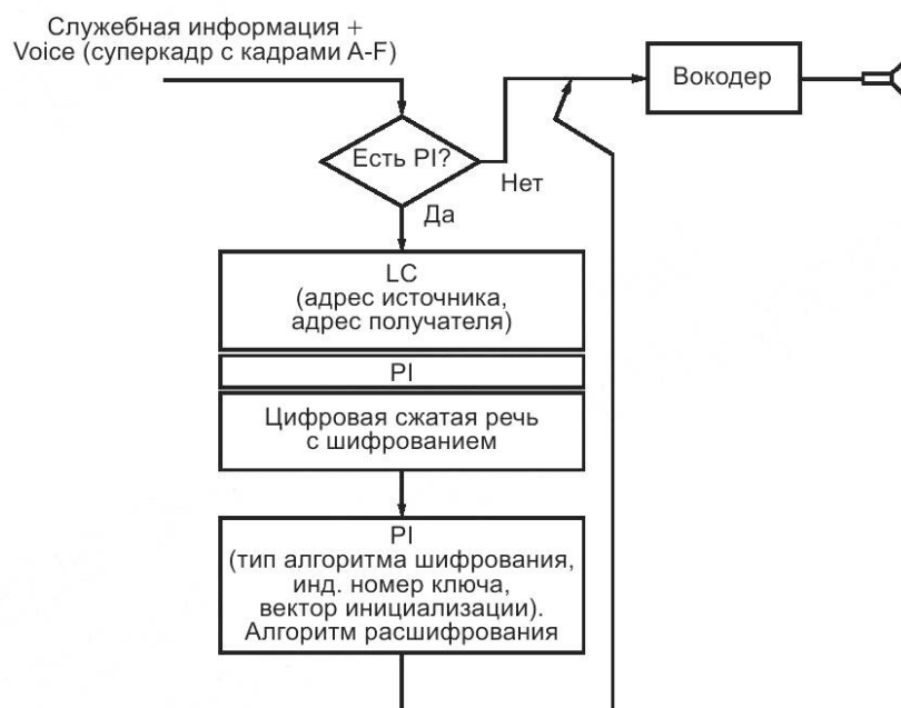
Рисунок 16 — Структурная схема расшифрования речевого сообщения в AC
