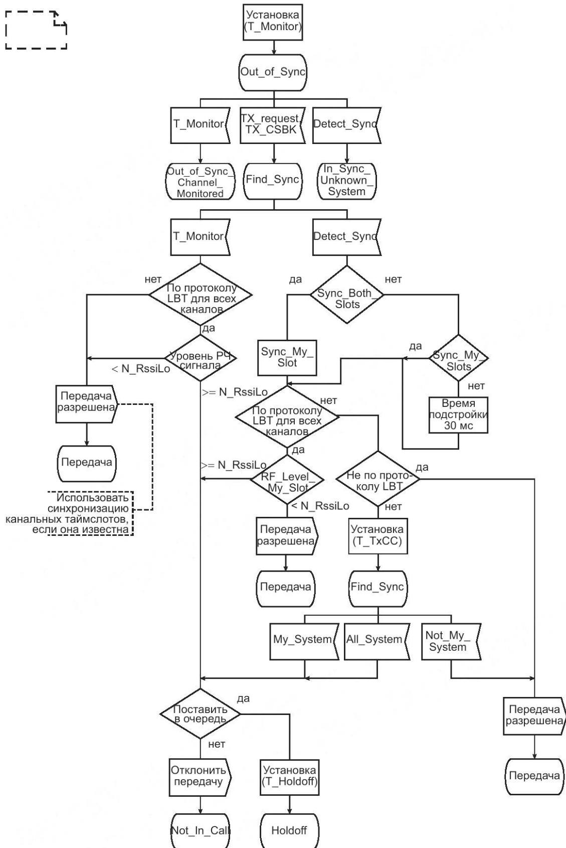
Рисунок 37 — SDL-диаграмма Out_of_Sync
