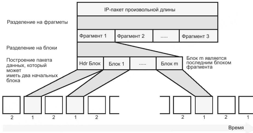
Рисунок 108 — Фрагментация IP-пакета
