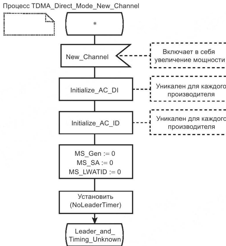
Рисунок 78 — SDL повышения мощности и смены канала
