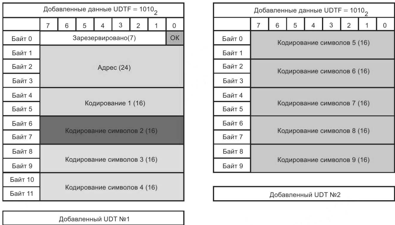
Рисунок Б.32 — Смешанный формат AD. Один адрес плюс шестнадцатибитные символы. От 4 до 9 символов
