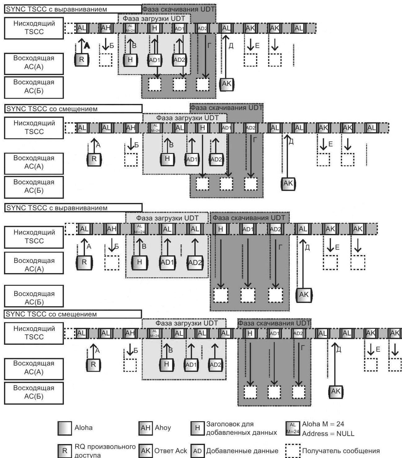
Рисунок 67 — Примеры передачи коротких данных с помощью UDT
