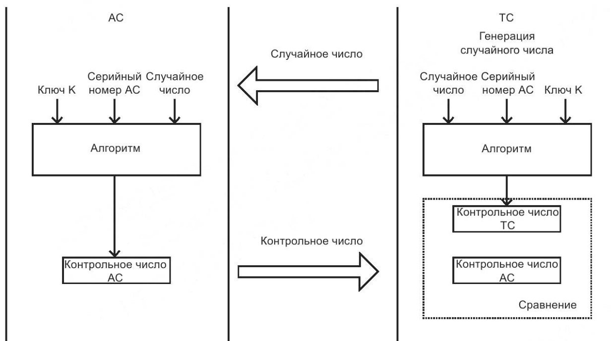
Рисунок 34 — Процедура аутентификации
