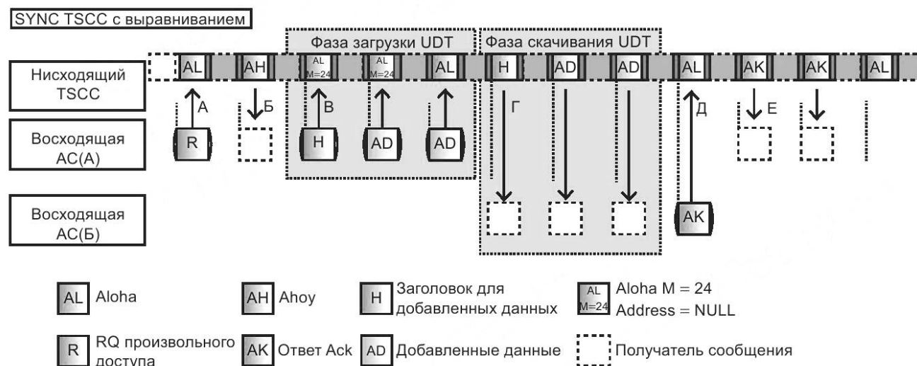
Рисунок 62 — Пример передачи данных при DGNA
