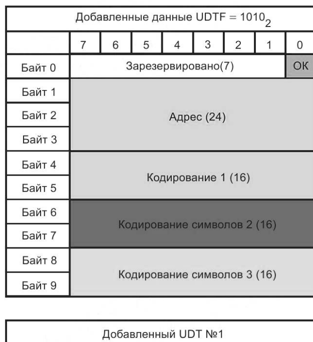
Рисунок Б.31 — Смешанный формат AD. Один адрес плюс шестнадцатитбитные символы. От 1 до 3 буквенных символов
