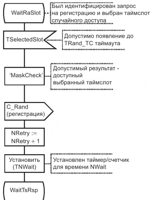
Рисунок 29 — SDL-диаграмма процесса регистрации с аутентификацией. Часть 1
