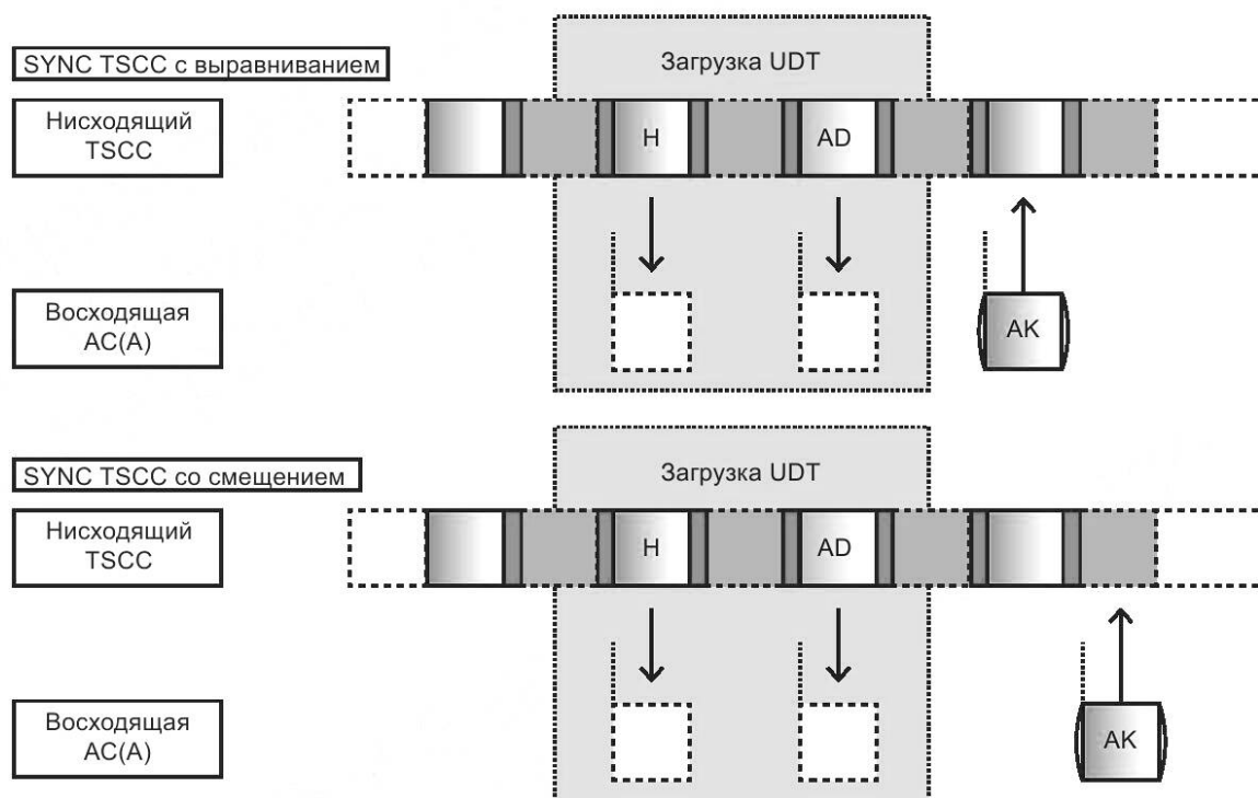
Рисунок 45 — Услуга передачи дополнительных данных пользователя в нисходящем направлении к АС от TSCC
