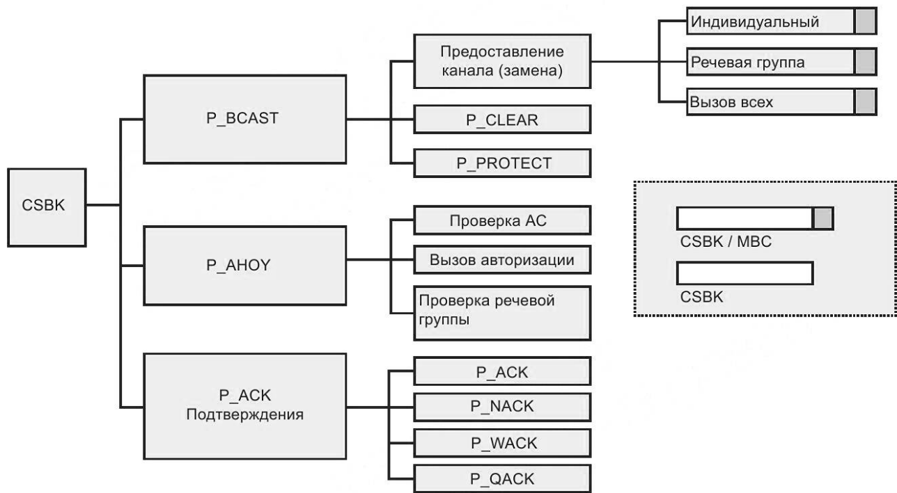
Рисунок 6 — Структура CSBK нисходящего рабочего канала
