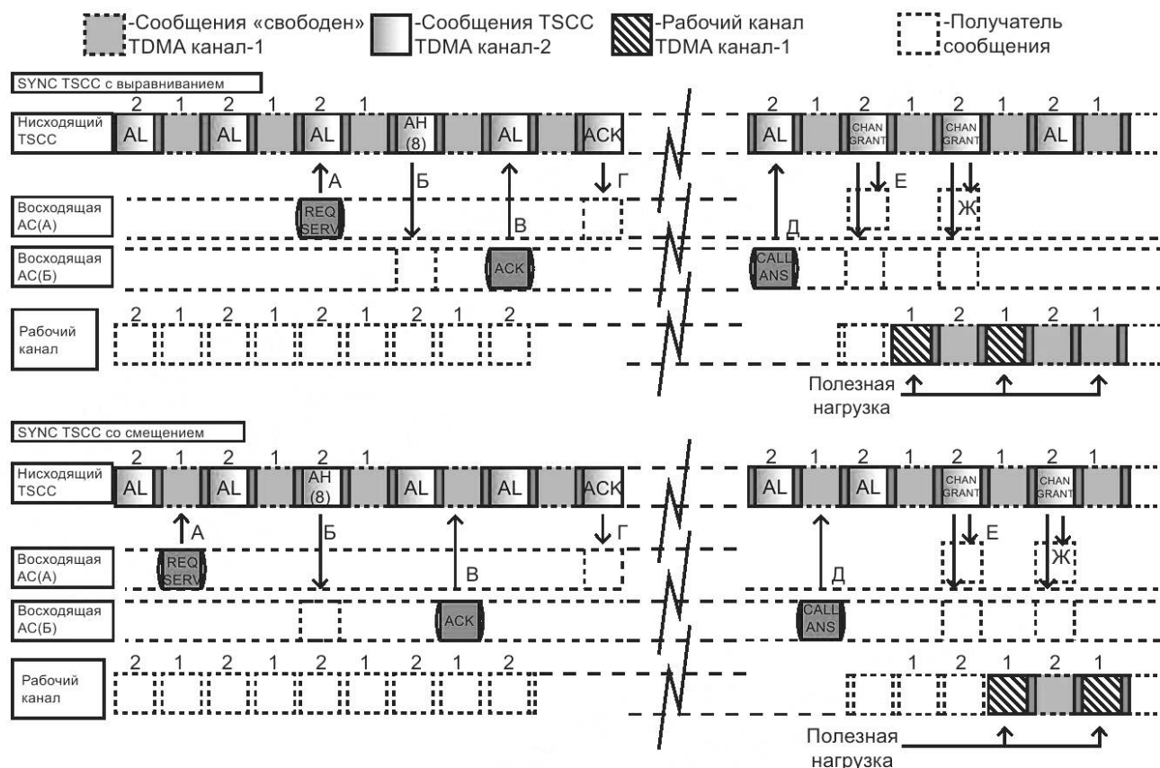
Рисунок 71 — Установление индивидуального вызова FOACSU
