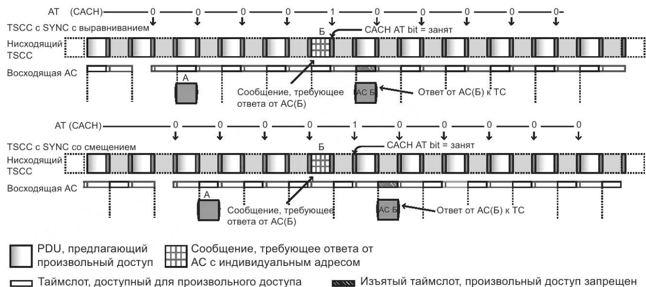
Рисунок 12 — Пример изъятия таймслотов
