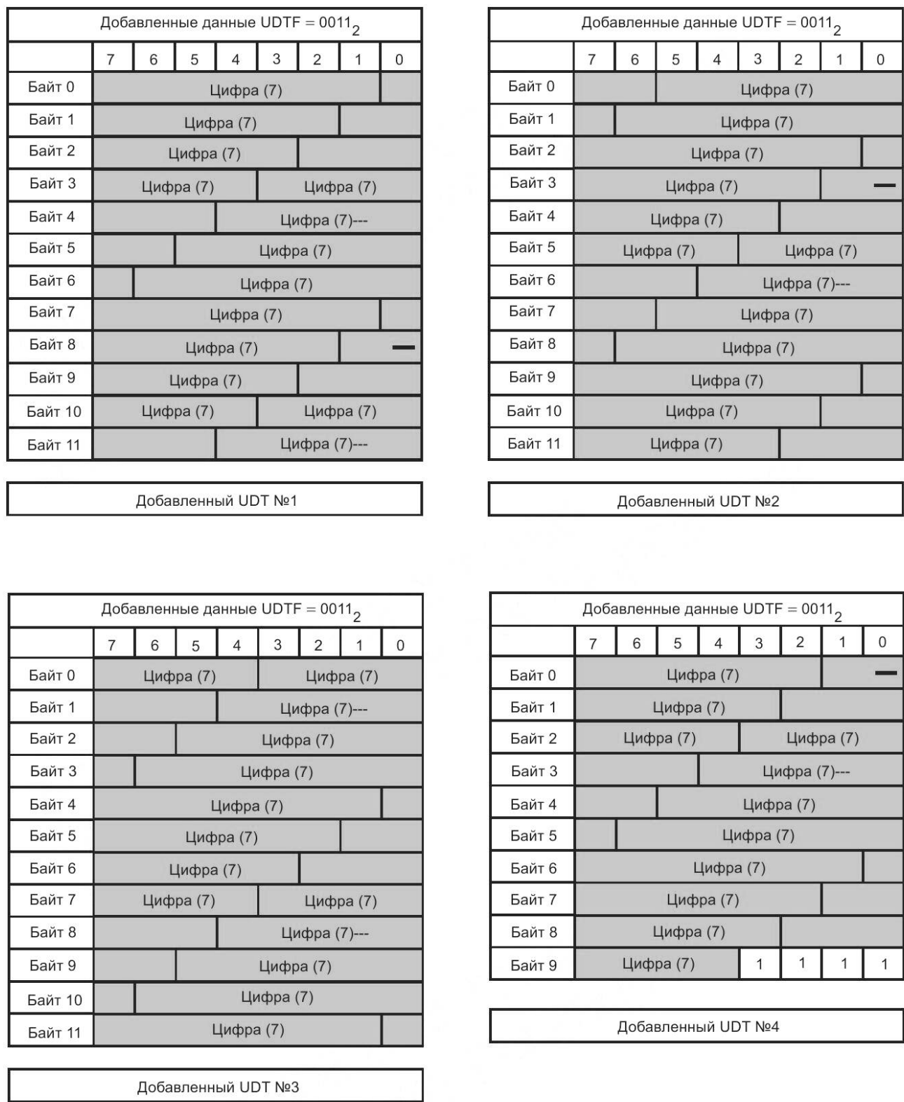
Рисунок Б.17 — Формат передачи унифицированных данных (7 бит ISO) от 39 до 52 символов
