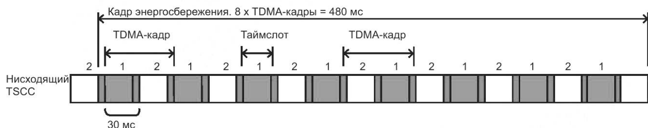
Рисунок 2 — Таймслоты и кадры TSCC
