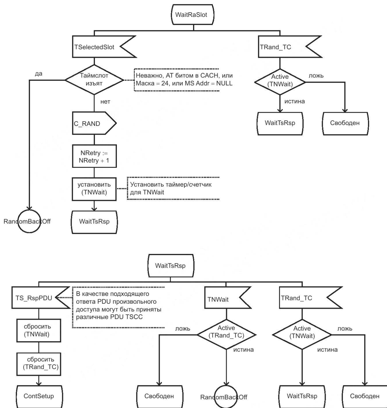
Рисунок 16 — SDL-процедура произвольного доступа
