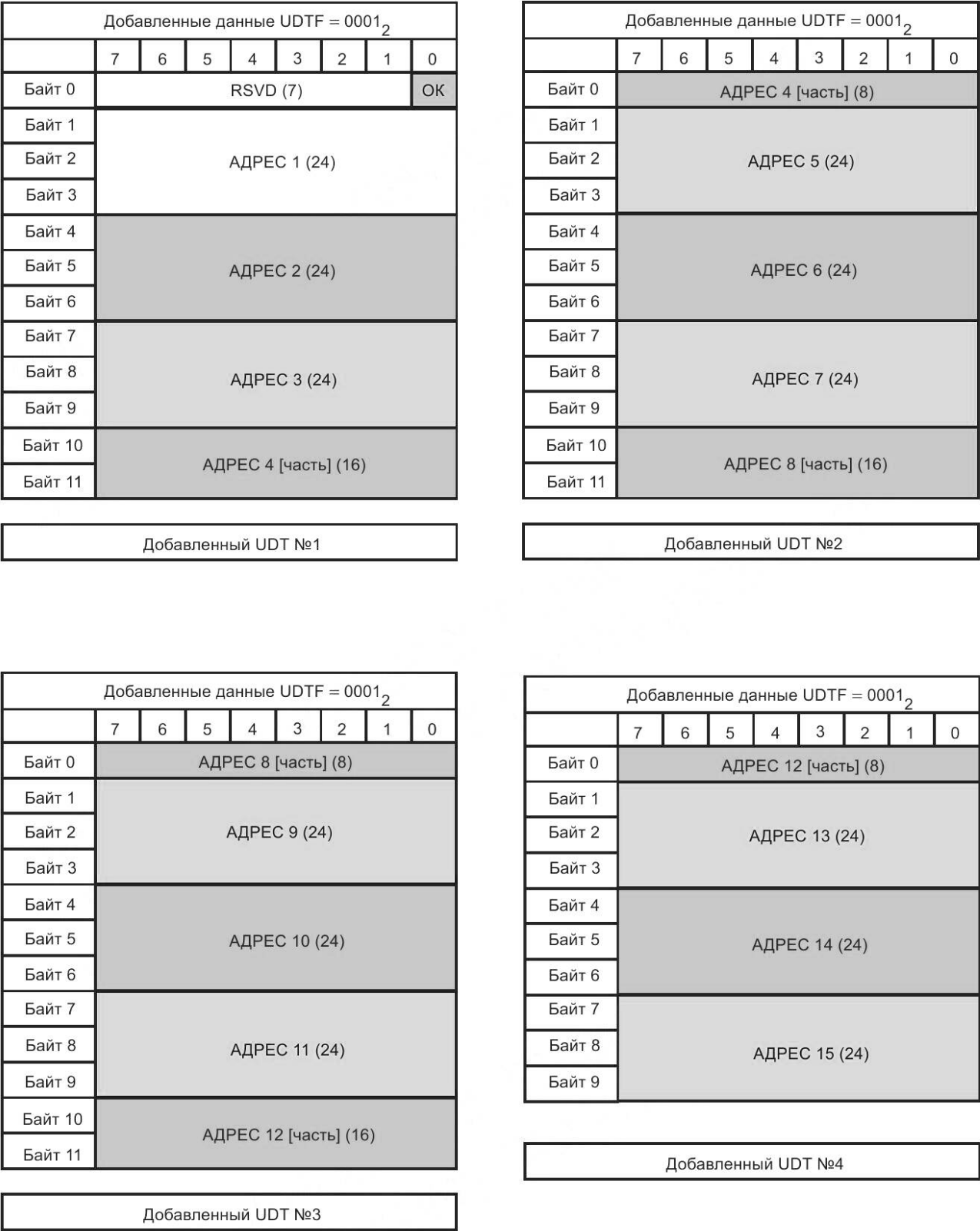
Рисунок Б.9 — Формат адреса AD (15 адресов)
