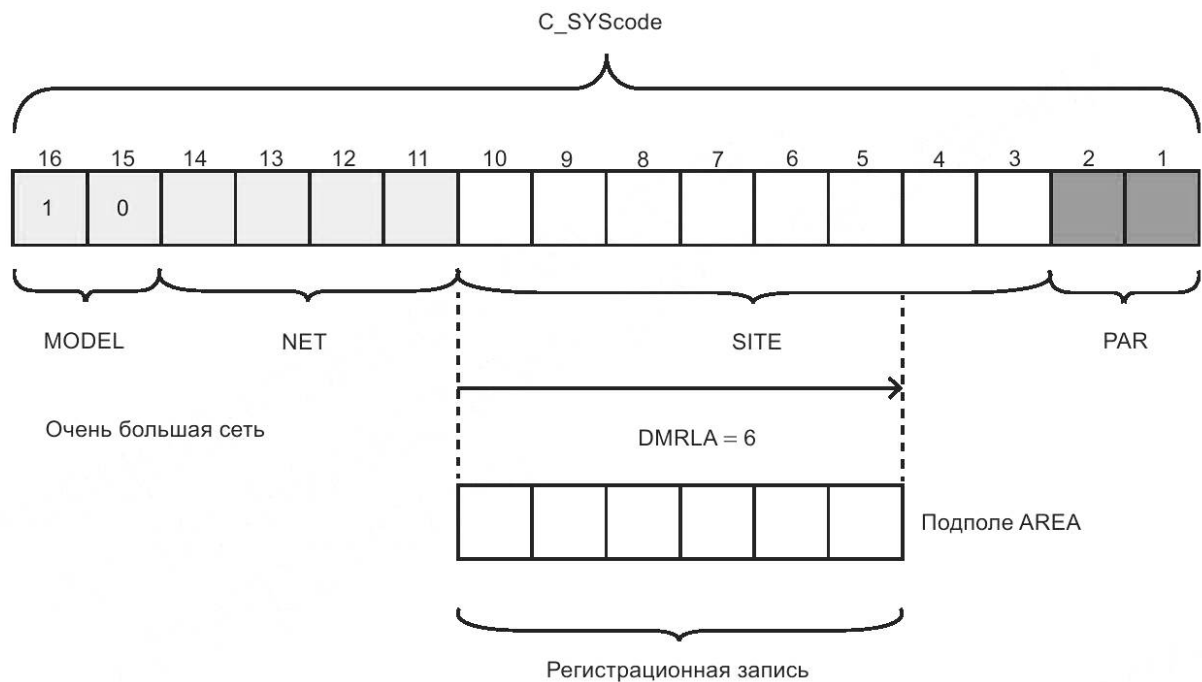
Рисунок 26 — Извлечение регистрационной записи из C_SYSCode
