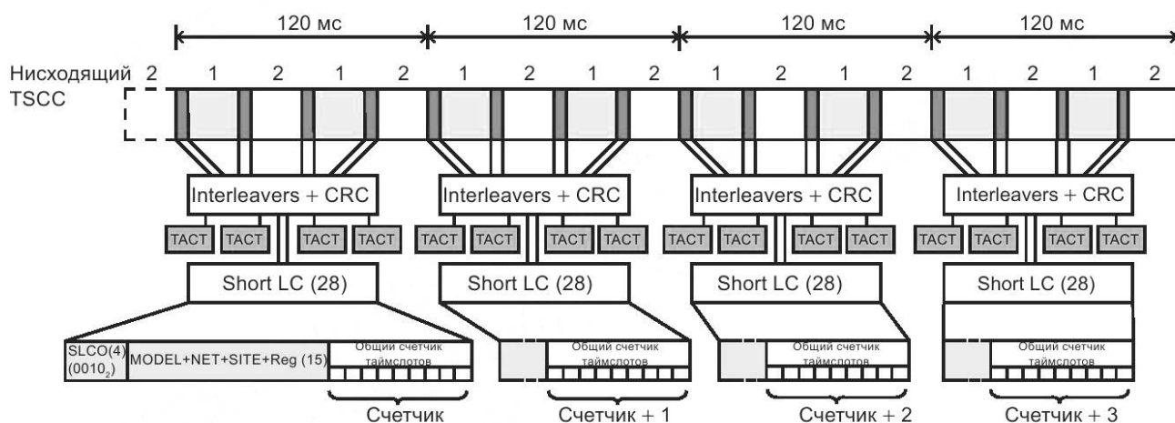
Рисунок 3 — Общий счетчик таймслотов
