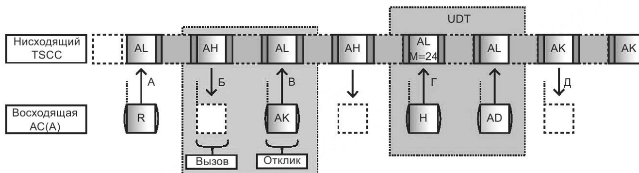
Рисунок 32 — Регистрация с подпиской/присоединением разговорной группы и аутентификацией
