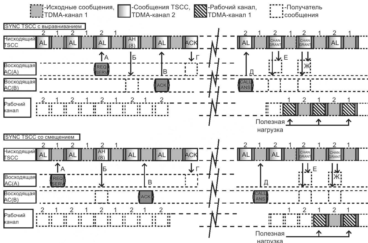
Рисунок 50 — Процедура ответа на вызов по принципу FOACSU
