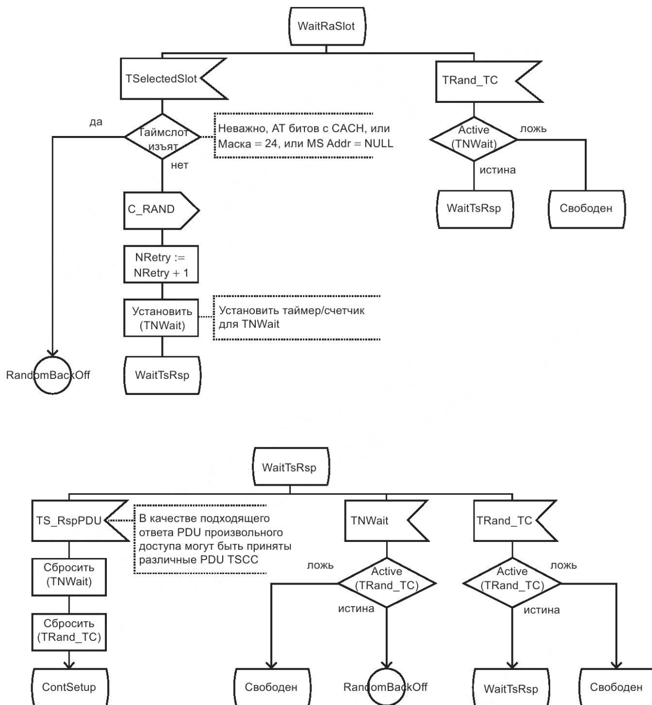
Рисунок 19 — SDL-процедура произвольного доступа в аварийных ситуациях
