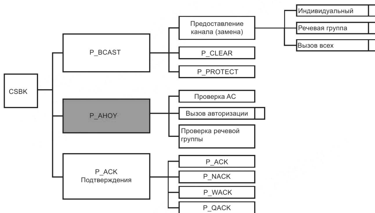
Рисунок 102 — PDU P_AHOY, передаваемый в рабочих каналах, в общей структуре и иерархии служебных сообщений
