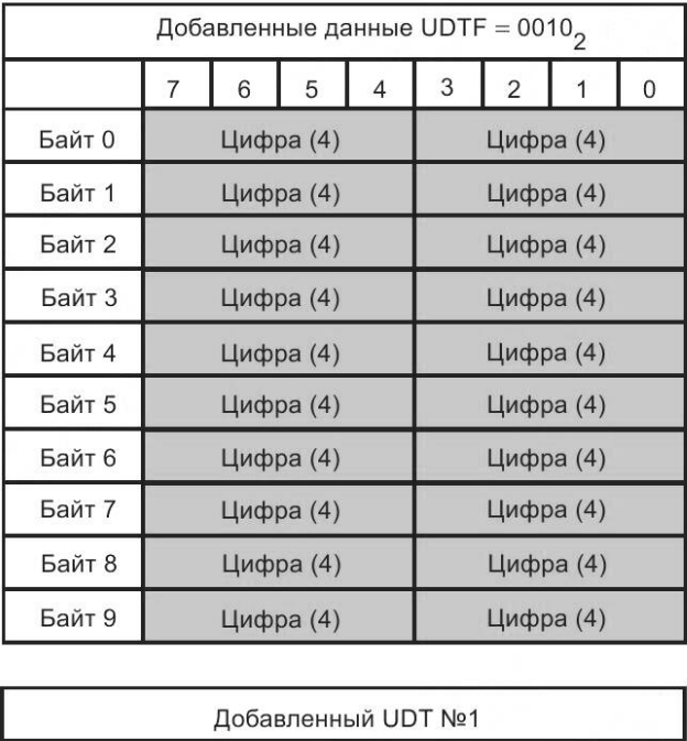
Рисунок Б.10 — Формат передачи унифицированных данных (BCD) от 1 до 20 цифр
