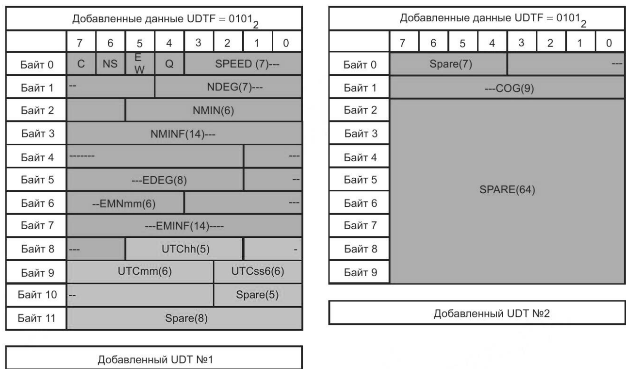
Рисунок Б.23 — Определенный длинный формат NMEA AD
