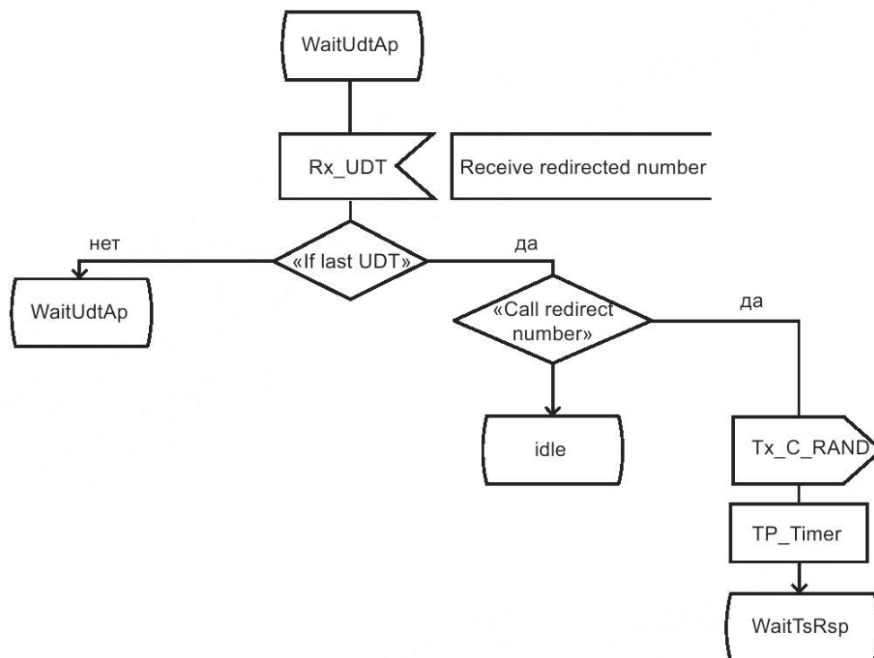
Рисунок 52 — SDL одноплочного установления речевого вызова OACSU. Часть 2
