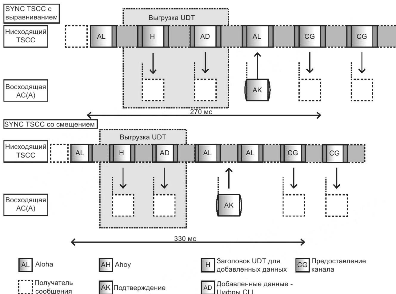
Рисунок 77 — Процедура UDT, передающая AD
