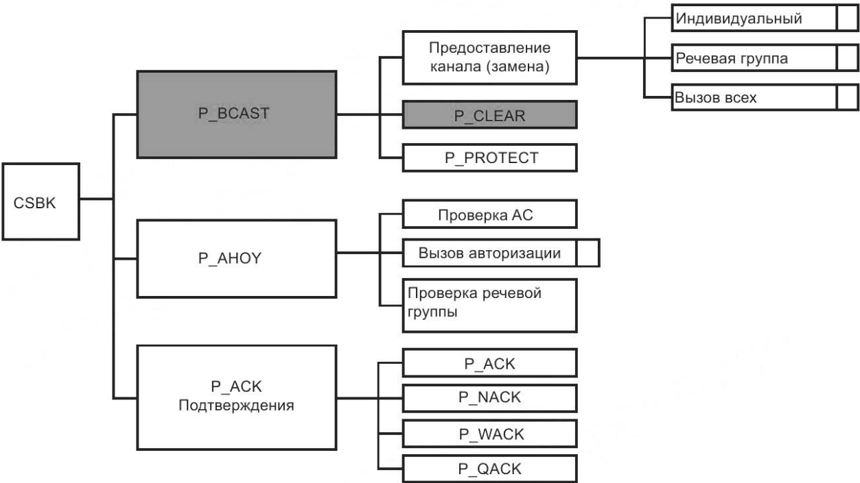
Рисунок 100 — PDU P_Clear, передаваемый в рабочих каналах в общей структуре и иерархии служебных сообщений
