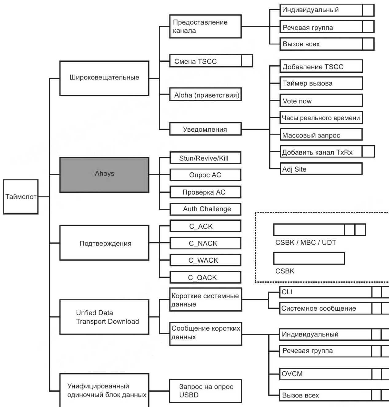
Рисунок 92 — PDU приветствия АНОУ в общей структуре и иерархии служебных сообщений в нисходящем направлении TSCC
