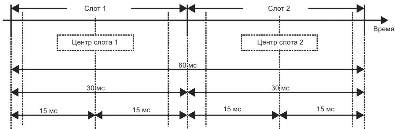
Рисунок 107 — Кадр TDMA
