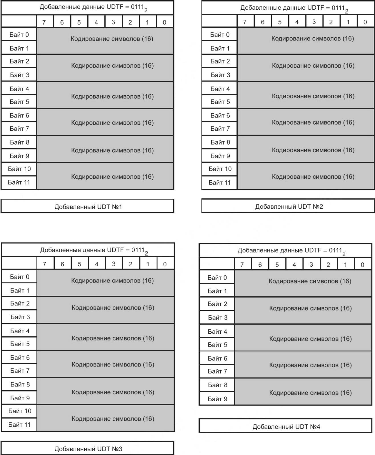
Рисунок Б.30 — Формат передачи унифицированных данных (шестнадцатибитный символ) от 18 до 23 символов
