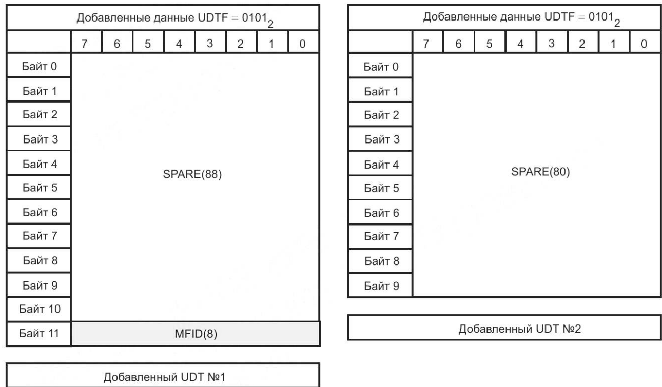
Рисунок Б.24 — Неопределенный длинный формат NMEA AD
