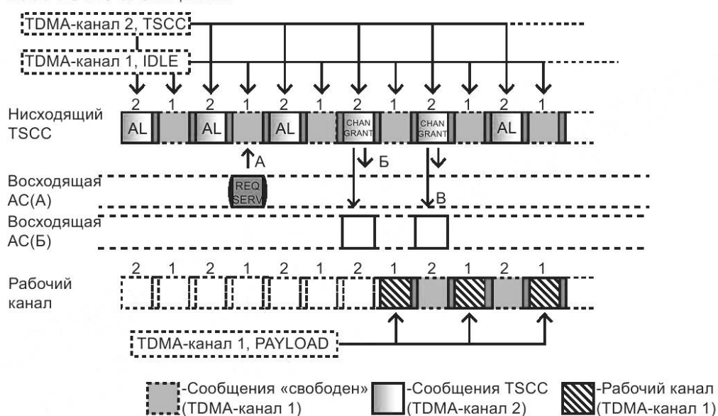
Рисунок 72 — Пример установления вызова разговорной группы
