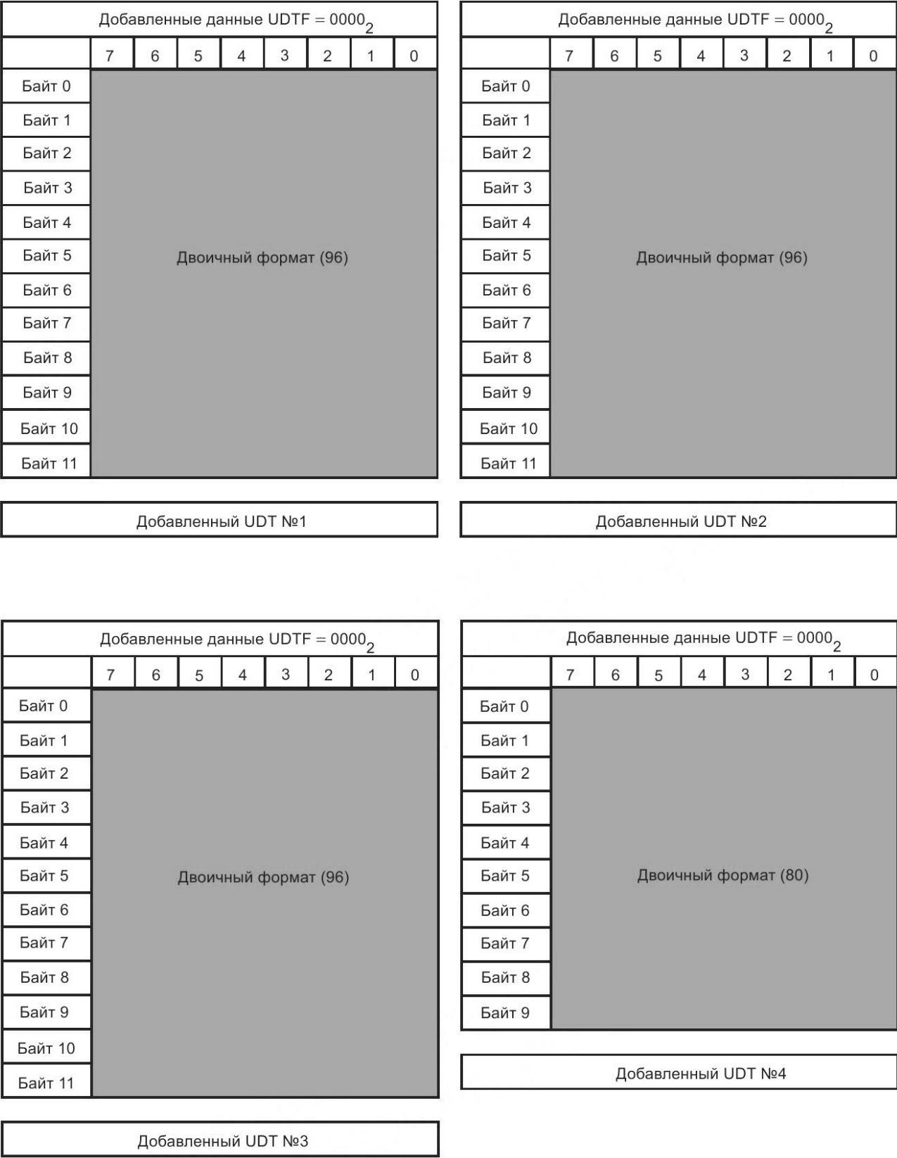
Рисунок Б.5 — Формат передачи унифицированных данных (двоичный) от 272 до 376 бит
