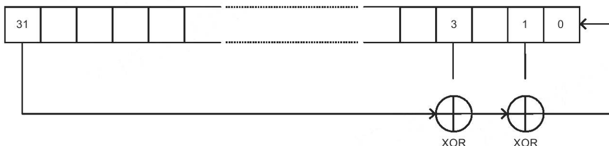
Рисунок 37 — Схема регистра LFSR
