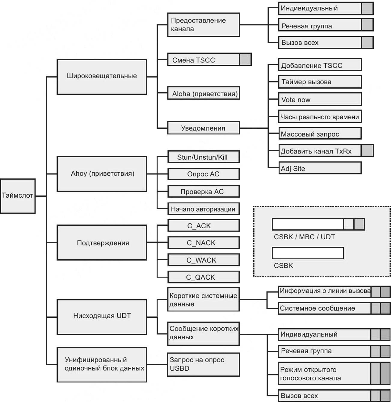
Рисунок 4 — Структура служебных сообщений CSBK/MBC/UDT/USBД, передаваемых TC в нисходящем TSCC
