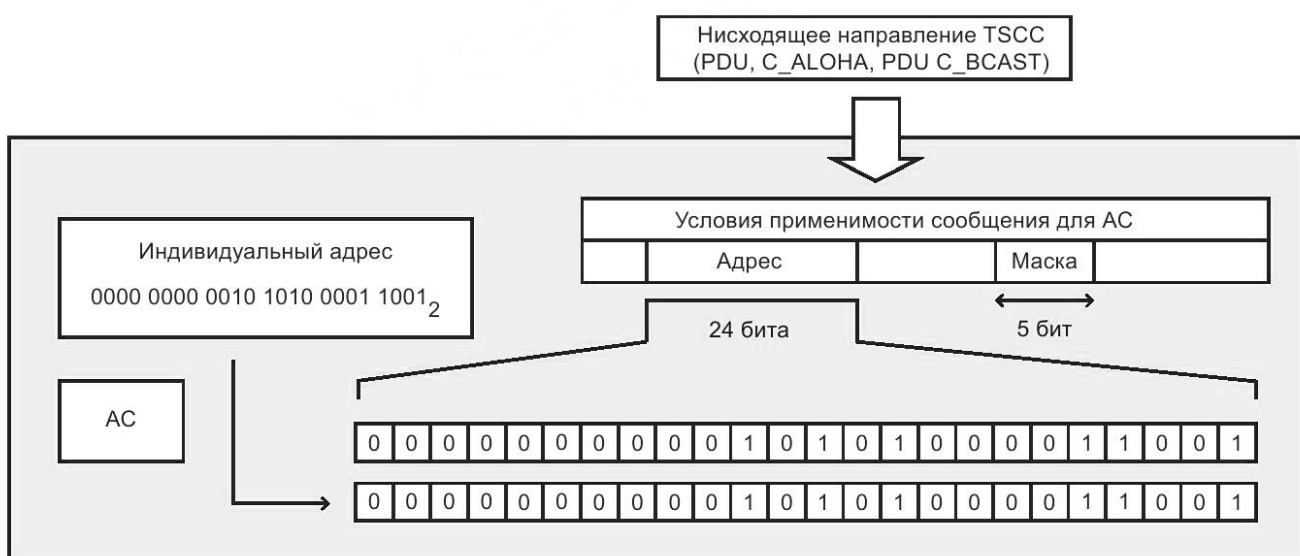
Рисунок 8 — Пример PDU, содержащего IE «Маска»
