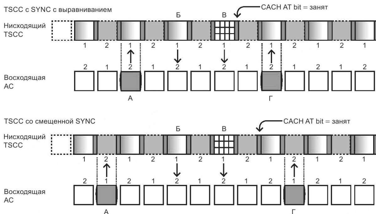
Рисунок 69 — Ключевые моменты для TSCC
