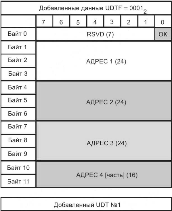
Рисунок Б.7 — Формат адреса AD (7 адресов)
