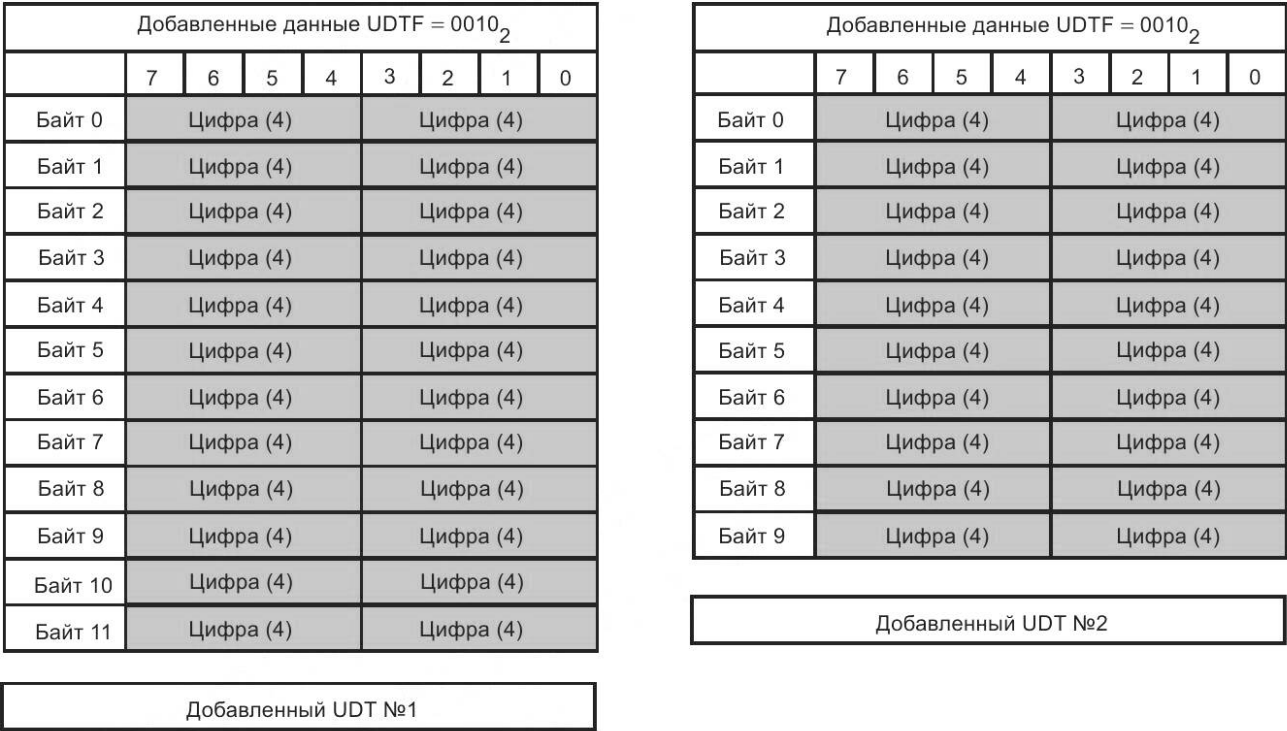
Рисунок Б.11 — Формат передачи унифицированных данных (BCD) от 21 до 44 цифр
