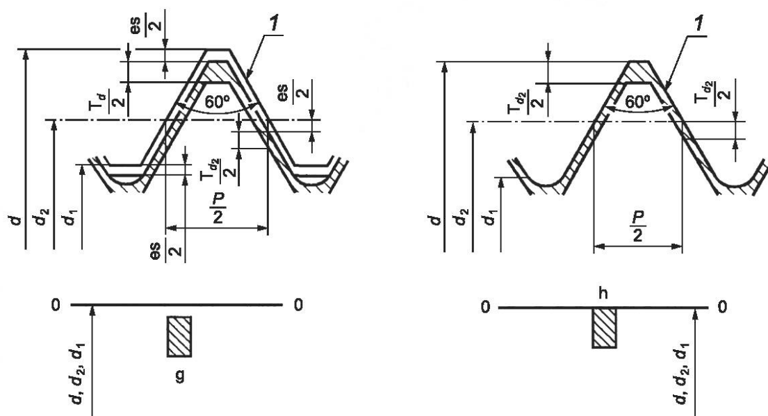
Рисунок 2 — Расположение полей допусков болтов с основными отклонениями g и h
