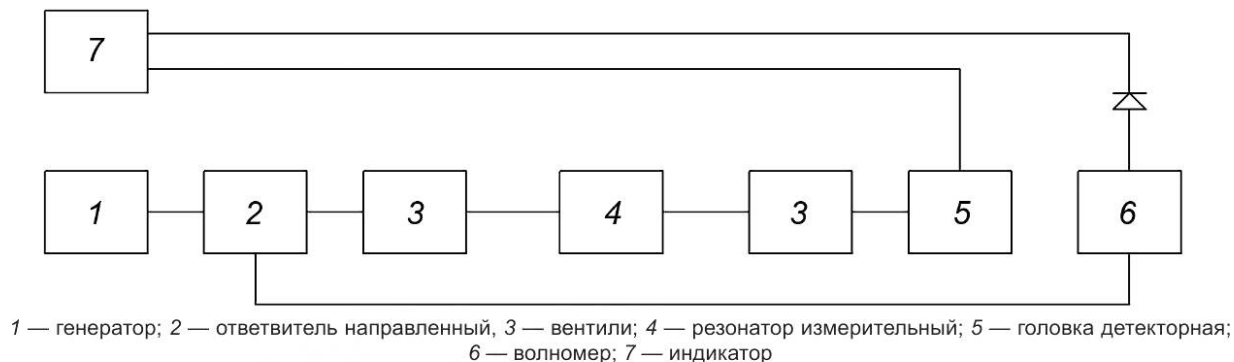
Рисунок 3 — Электрическая структурная схема
