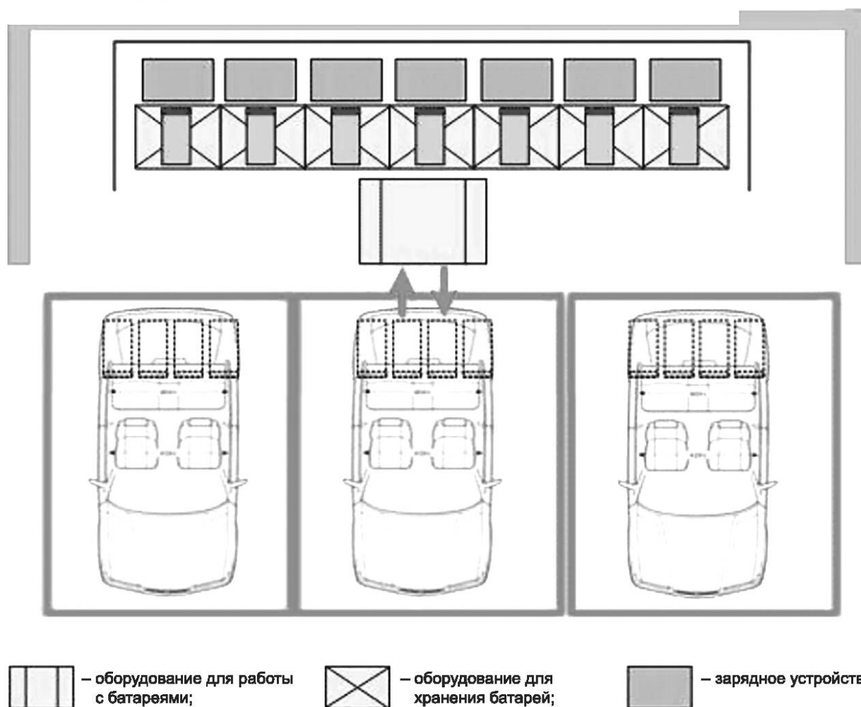
Рисунок В.3 — Полуавтоматизированная станция с задней заменой батареей
