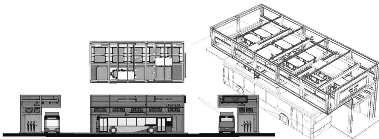
Рисунок В.2 — Схема автоматизированной станции с верхней заменой батарей
