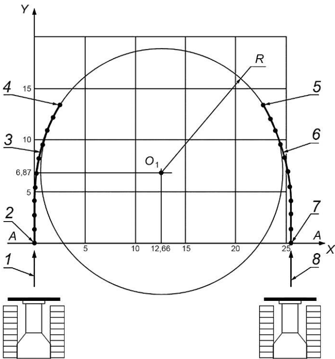
1, 8 — направление движения РВАЗДСМ гусеничного или колесного типа перед выездом на траекторию; 2, 7 — стартовые точки движения по траекториям; 3 — траектория поворота РВАЗДСМ направо; 4, 5 — финишные точки движения по траекториям; 6 — траектория поворота РВАЗДСМ налево; AA — стартовая линия
